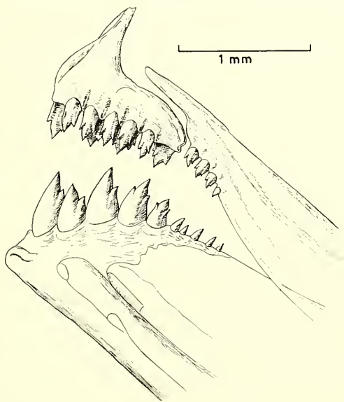
Fig. 5 : Mâchoires gauches, vue externe, de G. terofali (paratype ♀ No 22141,7; demi-schématique).
