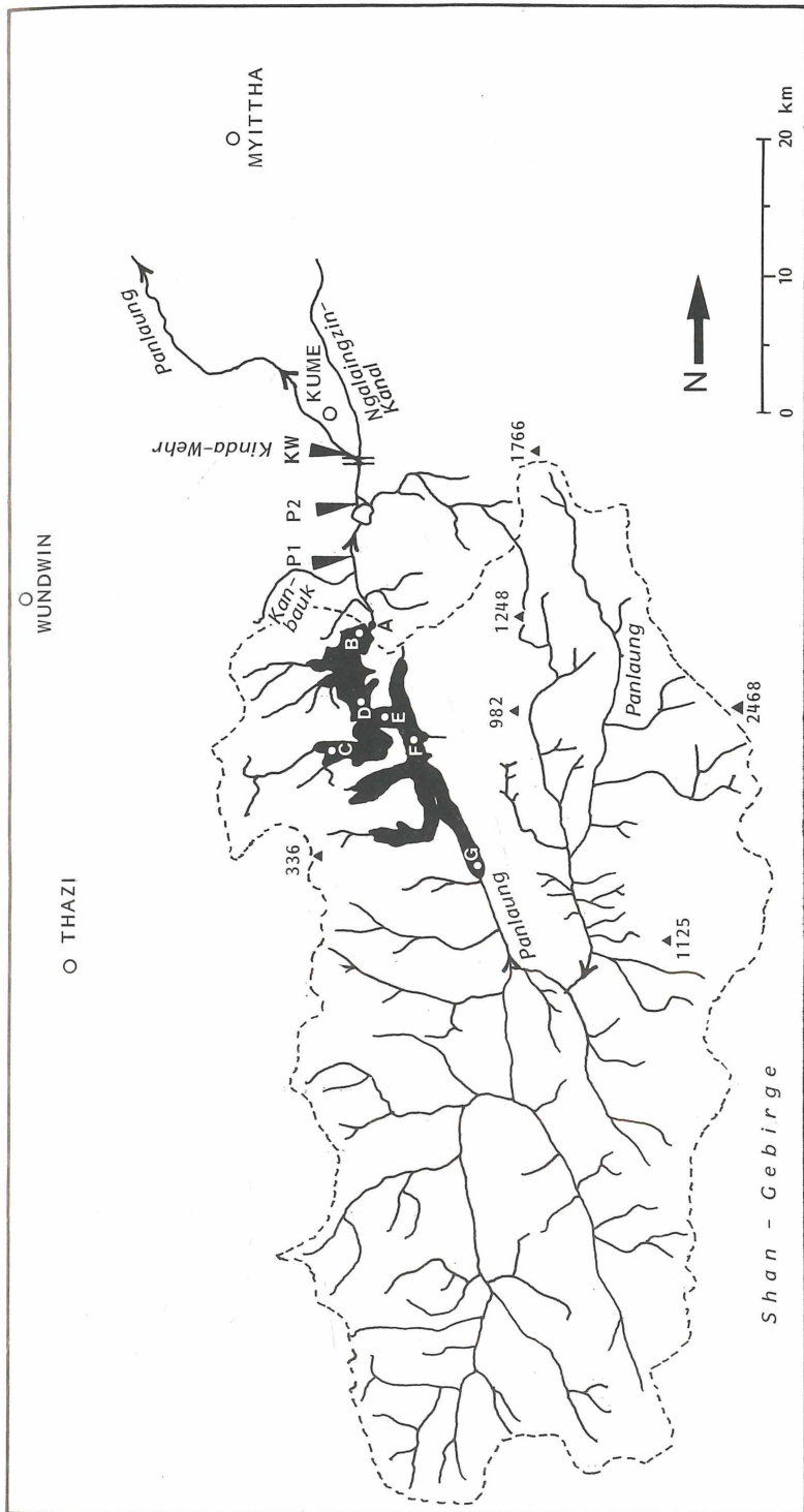
Abb. 1. Karte des Kinda-Stausees (schwarz) und seines Einzugsgebietes. – Es bedeuten: A–G, P1–P2, KW = Probenentnahmestellen (vgl. dazu Tabelle 1). Die Zahlen beziehen sich auf Gebirgshöhen in m.
