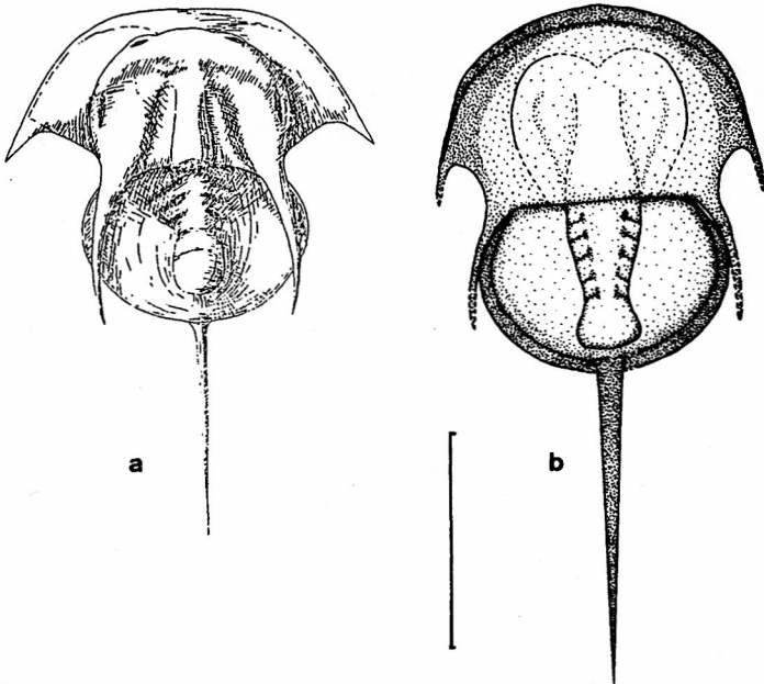
Abb. 5 Rekonstruktion der zwei Palatinaspis -Arten. a) Palatinaspis fritschi aus dem Stefan C der Halleschen Mulde. – Nach W. & R. REMY 1959. b) Palatinaspis beimbaueri n.g. et n.sp. aus dem Unter-Rotliegenden von Niedermoschel/Pfalz. – Maßstab = 1 cm.
