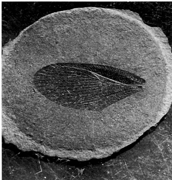
Abb. 2 Vorderflügel von Phyloblatta sp. (Schabe) aus dem Unter-Rotliegenden von Niedermoschel/Pfalz; x 3 (fot. S. Tränkner). – Paläontol. Mus. Nierstein, SSN 11 NM 2.
