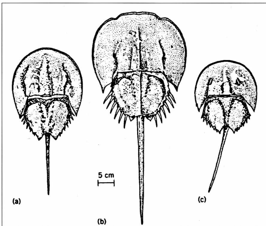
Abb. 3 Gegenüberstellung von adulten Panzern rezenter Limuliden: (a) Limulus polyphemus , (b) Tachypleus tridentatus , (c) Carcinoscorpius rotundicauda . – Aus SHUSTER 1982a.
