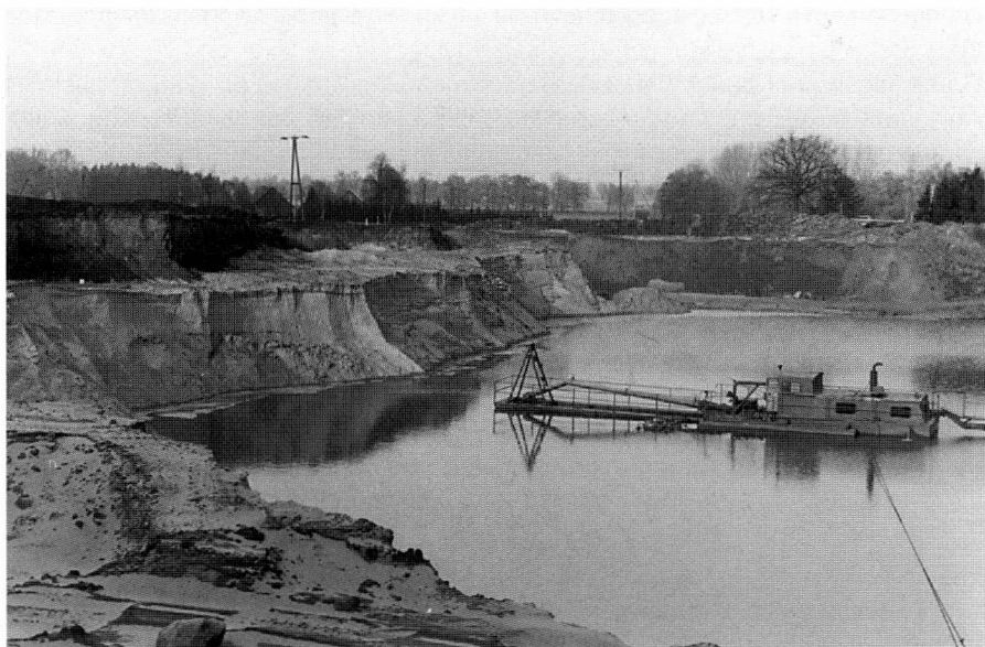
Abb. 2 Saalezeitliche Grundmoräne über Schmelzwassersanden in der Westwand der Sandgrube Bockbreder (Länge der Grubenwand ca. 150 m)
