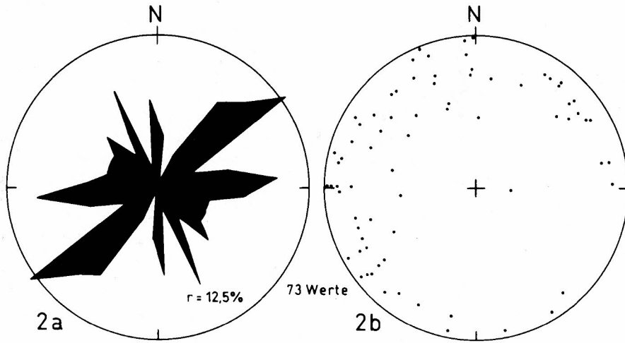
Grundmoräne, unterer Teil
