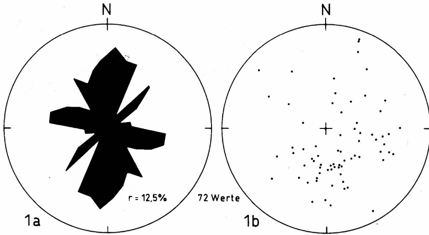
Grundmoräne, oberer Teil
