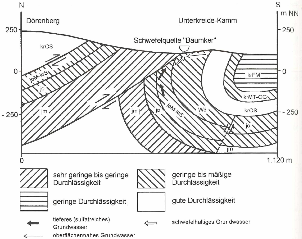
Abb. 8 Hydrogeologischer Schnitt im Bereich der Schwefelquelle „Bäumker“
