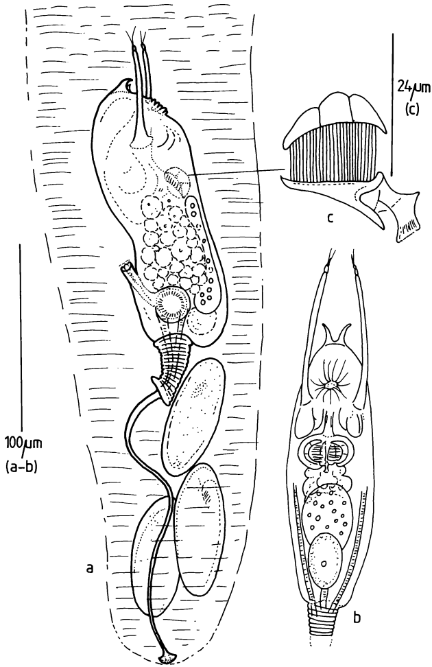
Abb. 11: Ptygura linguata Edmondson, 1939: a – kontrahiert, lateral; b – Körper ventral, c – Trophi, lateral.
