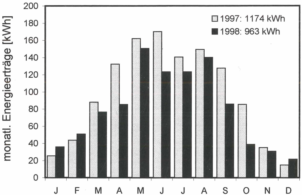
Abb. 4: Monatliche Erträge der Photovoltaikanlage 1998 (in kWh) verglichen mit den Werten von 1997.
