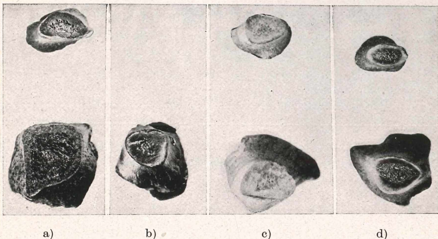
Abb. 7. Querschnittsbilder durch Ulna (obere Reihe) und Tibia (untere Reihe) von a) Miophoca vetusta , Torton, Sandberg; b) Phoca vindobonensis , Sarmat, Nußdorf; c) Phoca vitulina , rez. (Paläontolog. u. Paläobiolog. Inst.); d) Phoca hispida , rez. (Paläontolog. u. Paläobiolog. Inst.). Die Schnitte wurden an allen Knochen in gleicher Höhe angefertigt. b) und c) sind osteosklerotisch.
