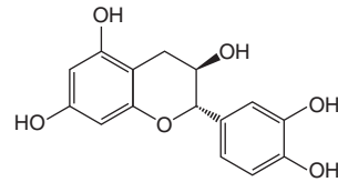
Abb. 1. Strukturformel von (-)-Catechin (Flavan-3-ol).
