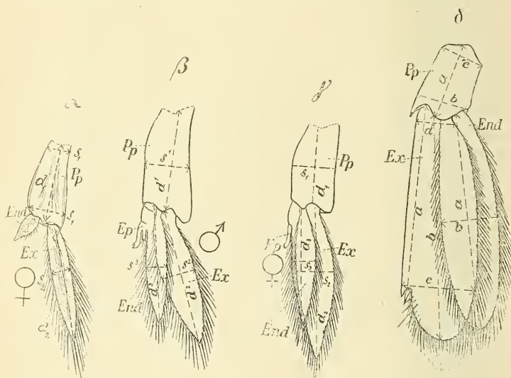
Obr. 30. Pleopodity sp. At. d. J. označením dimensí. α. pár 1.; β a γ. pár 2.; δ. pár 6. End. , Endopodit; Ex. , exopodit; Ep. , epipodit; Pp. , propodit.
