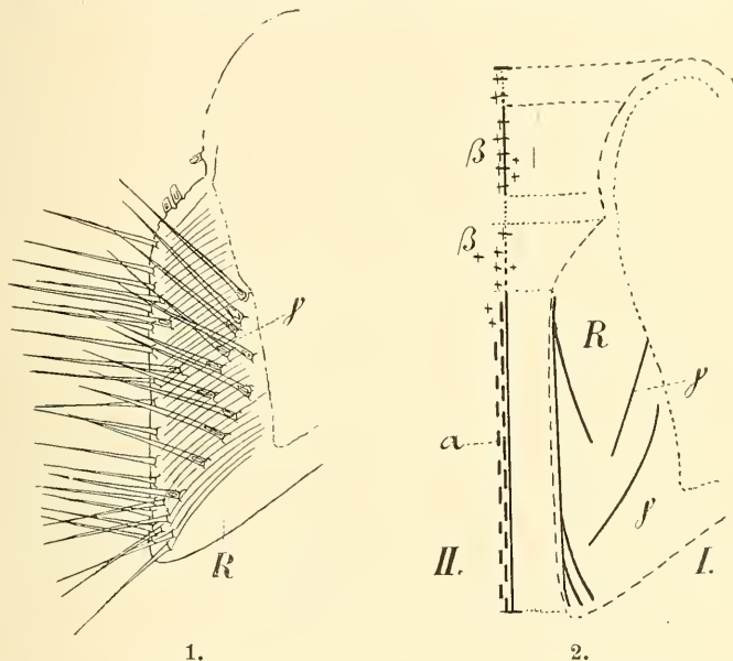
Obr. 21. 1. Sestavení štětín \gamma na chitinové obrubě (R) kus. lamelly 2. maxillipedu. 2. Diagram téhož. Označení štětín (vzhledem k obr. 20., 21. [1.]) \alpha |, \beta +, \gamma -; I. Plocha spodní (od těla), II. svrchní (k tělu).
