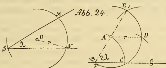
Abb. 24. Verbindung von IV_2 mit IXb . E = 15 ; 5 Kreise, 1 Gerade.
