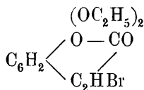
Monobromdiäthyldaphnetin
