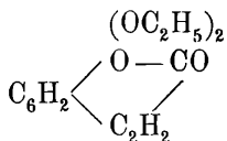
Diäthyldaphnetin
