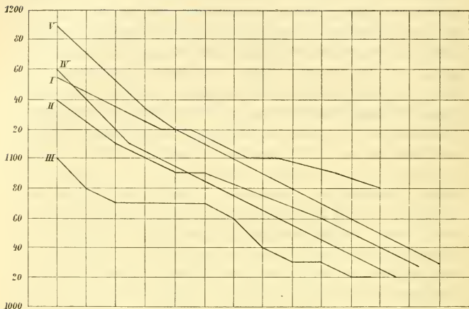
Fig. 4. Labrador-Diopsid (Mineralmenge).
