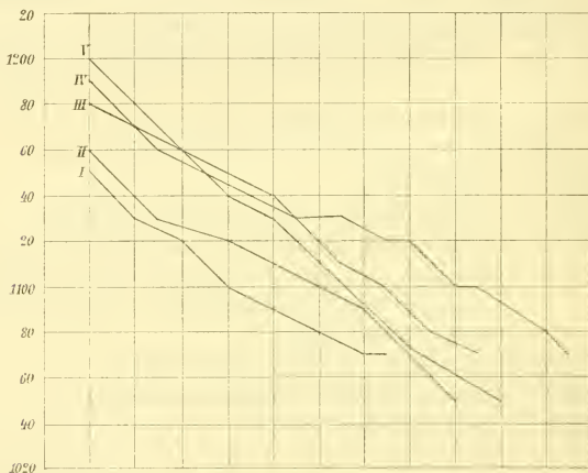
Fig. 6. Labrador-Diopsid (chemische Mischungen).
