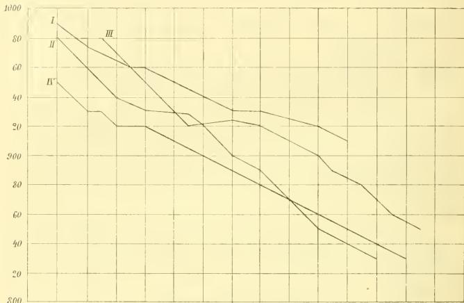
Fig. 2. Ägirin-Eläolith (Mineralgemenge).
