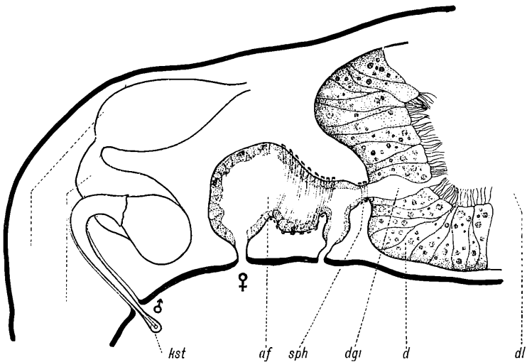
Fig. Promacrostomum paradoxum nov. gen. nov. spec.; Organisationschema des Genitalapparates.
