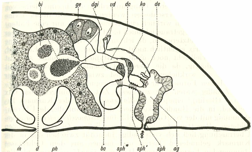
Fig. 23. Olisthanella truncula (O. Schmidt); Organisationsschema des Genitalapparates.
