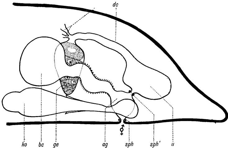
Fig. 6. Dalyellia minima nov. spec.; Organisationschema des Genitalapparates.
