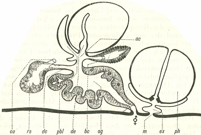
Fig. 21. Castrada ochridense nov. spec.; Organisationsschema des Genitalapparates.
