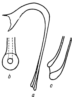
Fig. 4. Promacrostomum paradoxum nov. gen. nov. spec.; Kutikularstilet, a = Totoansicht, b und c = Ende des Kutikularstilettes in Vorder- und Seitenansicht.
