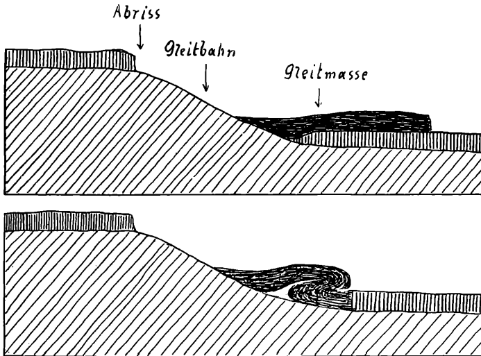
Fig. 1. Einfache, unten freie Gleitung.
