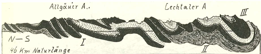
Fig. 10. I = Allgäudecke. Gestrichelt = mittlere untere Trias II = Lechtaldecke Schwarz = Hauptdolomit III = Inttaldecke Punktsaum — Kössener Sch. mit Krabachjochdecke Punktiert = Jura + Kreide + Tertiär
