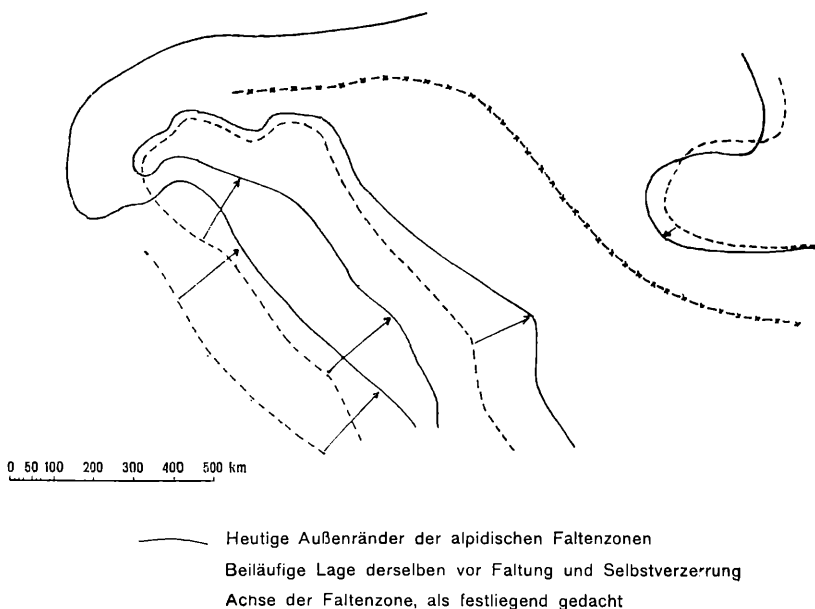
Abb. 5. Versuch einer Rekonstruktion der Selbstverzerrung der alpidischen Faltenzungen.
