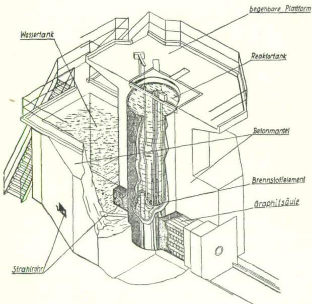
Abb. 1: Der Reaktor des Atominstutts der österreichischen Hochschulen.
