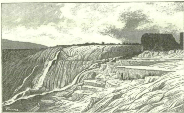
Die Kalksinterterrassen der Quellen von Hierapolis. (Pambuk-Kalessi.)
