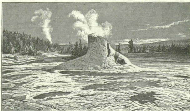
Die Sinterkegelröhre des Giant-Geysir.
