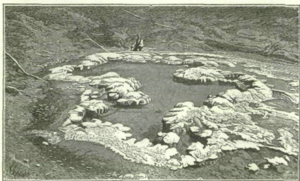
Sinterkranz des Deluge-Geysir.
