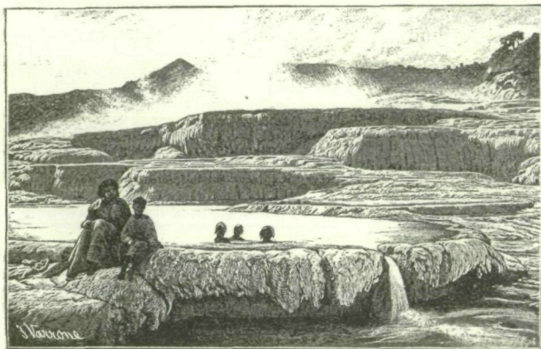
Eine Partie der Kieselsinterterrassen der Tetarata.
