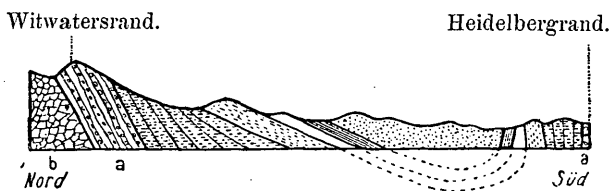
Fig. 9. Schnitt durch das Witwatersrand-Goldfeld.
