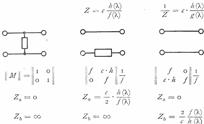
Abb. 2. Schaltungen, Kettenmatrizen und Brücken-Reaktanzen ausgearteter symmetrischer Vierpole
