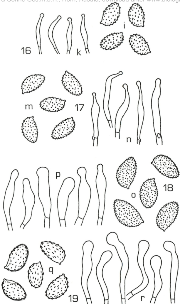
Fig. XIII. 16. Ph. primulina (BERK.) HK. (K, holotype): i. spores. — k. cheilocystidia. 17. Ph. subattenuata SINGER (LIL, B 2372; holotype): m. spores. — n. cheilocystidia. 18. Ph. odorata HK. (ZT, 73/313; holotype): o. spores. — p. cheilocystidia. 19. Ph. festiva (FR.) HEIM (ZT, 74/303): q. spores. — r. cheilocystidia.
