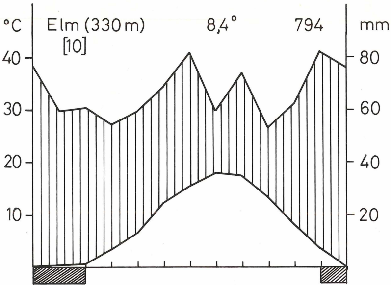
Abb. 1: Klimadiagramm für Elm
