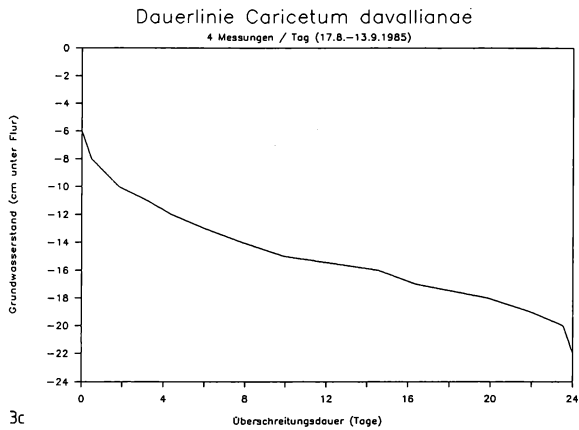
Abb. 3: Grundwasserdauerlinien des Caricetum davallianae nach Abb. 2 mit unterschiedlicher Meßpunktdichte. 3a: 14tägiger Meßsturnus; 3b: 2tägiger Meßsturnus; 3c: 4 Messungen/Tag.
