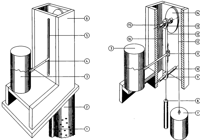
Abb. 1: Pegel-Meßgerät; Außen- und Innenansicht.
