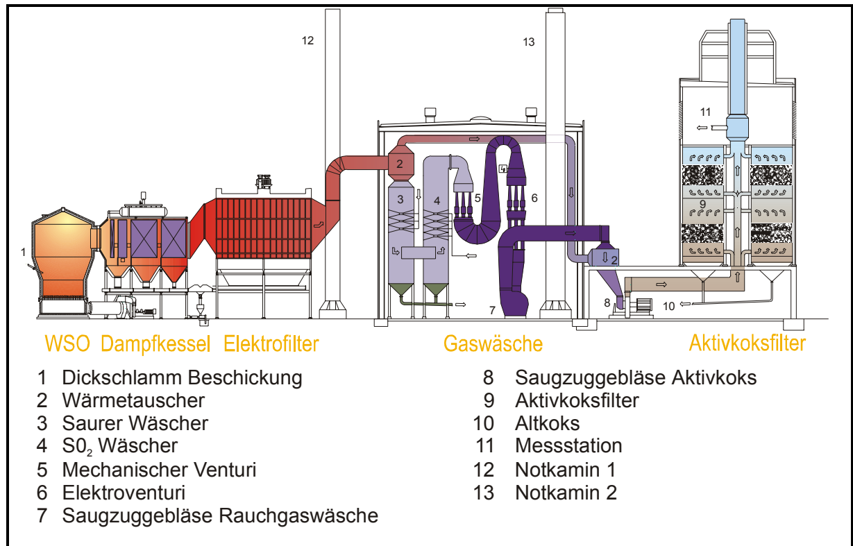
Abbildung 9: Fließbild Wirbelschichtöfen
