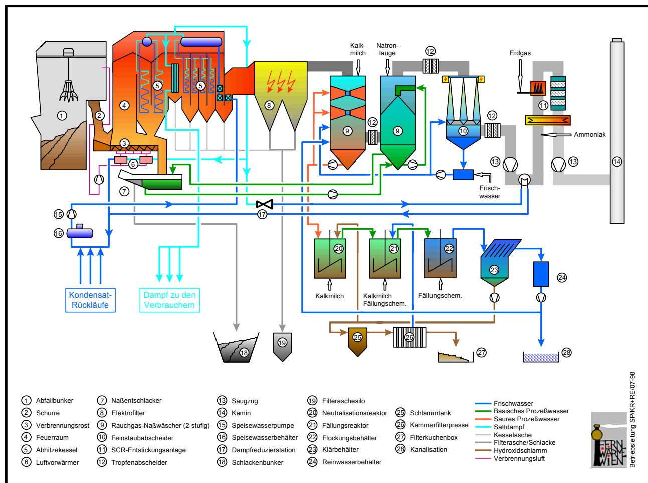
Abbildung 3: Fließschema der MVA Flötzersteig
