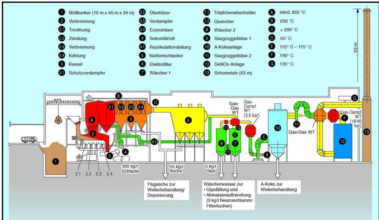
Abbildung 6: Verfahrenschema der Müllverbrennungsanlage Wels, Linie 1 (WACHTER 2000)
