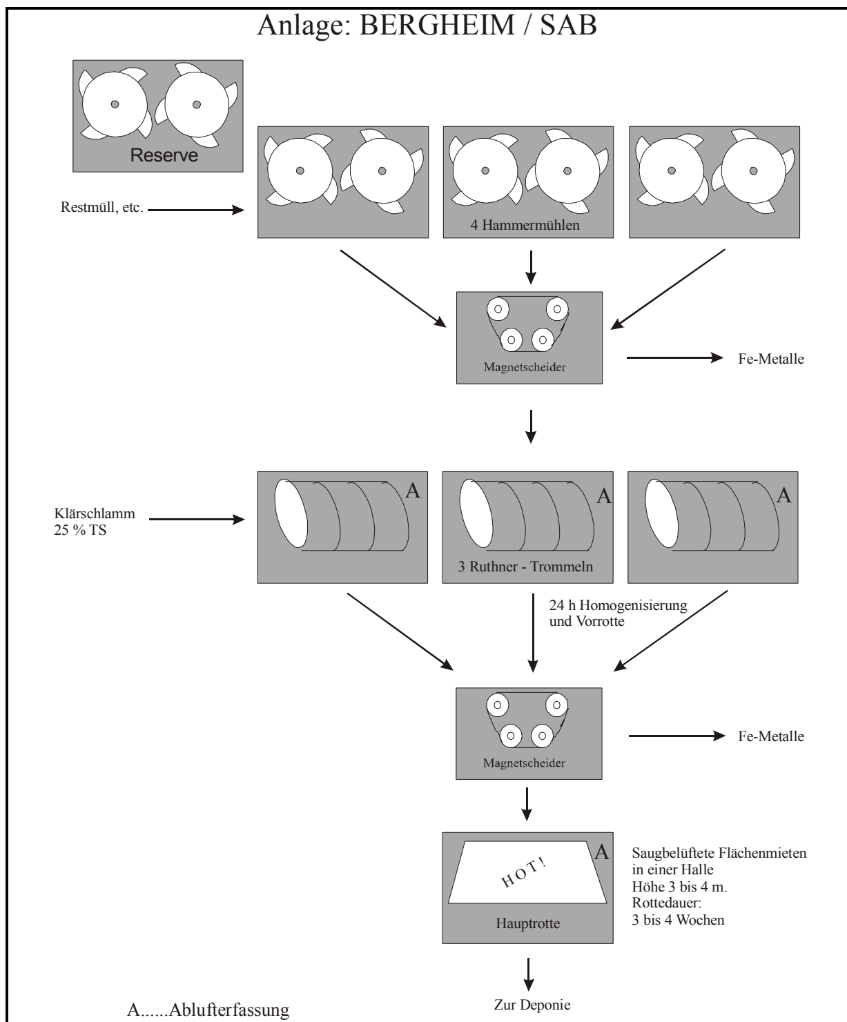
Abbildung 24: Fließbild der Anlage Siggerwiesen
