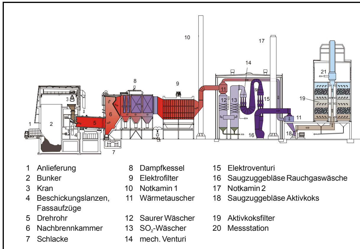
Abbildung 11: Fließschema Drehrohr
