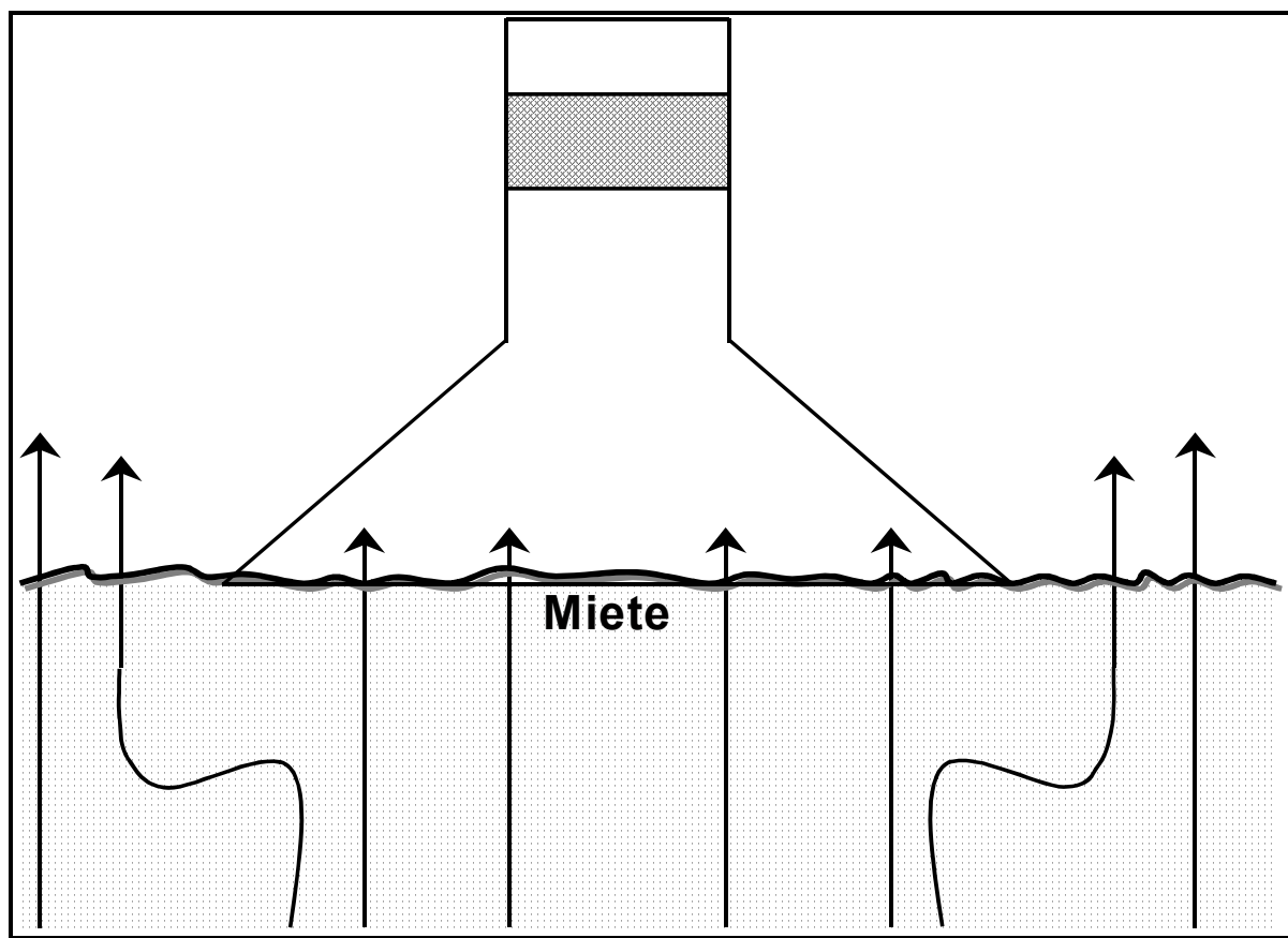
Abbildung 12: Prinzip der Probenahme der Abluft bei einer Freilandrotte (eigene Grafik)
