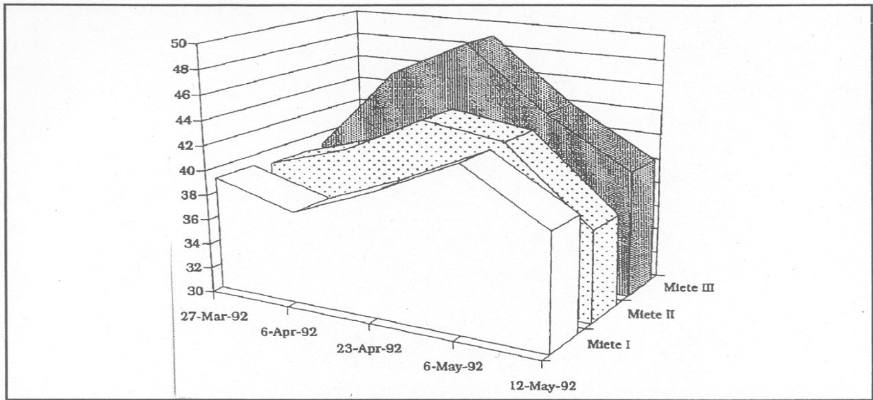
Abbildung 14: Pb gesamt in mg/kg TS (FORSTINGER, 1997)
