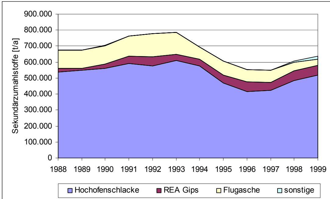
Abbildung 13: Einsatz an Sekundärzumahlstoffen in der österreichischen Zementindustrie 1988-1999 [Daten aus: HACKL & MAUSCHITZ, 1995, 1997, 2001]
