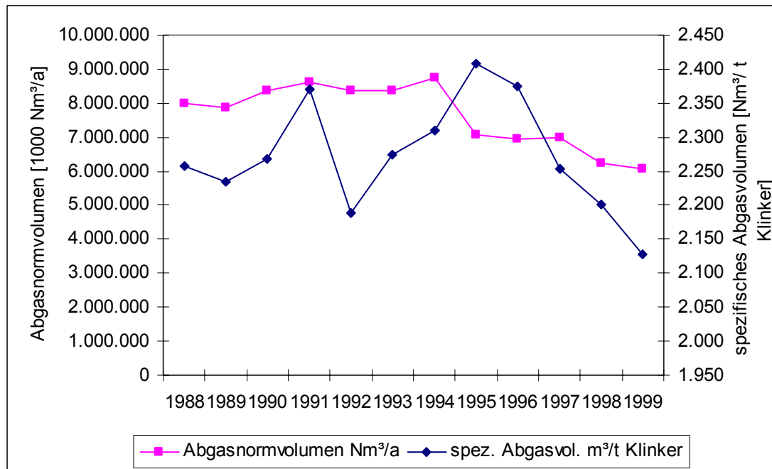
Abbildung 14: Gesamtes und spezifisches Abgasnormvolumen österreichischer Zementwerke der Jahre 1988 bis 1999 [Daten aus: HACKL & MAUSCHITZ, 1995, 1997, 2001]
