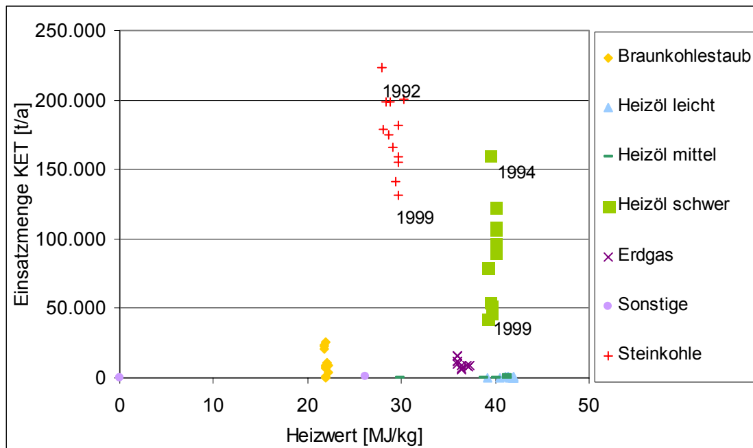
Abbildung 5: Heizwerte konventioneller Energieträger und die eingesetzten Mengen der jeweiligen Brennstoffe (1988-1999) [Daten aus: HACKL & MAUSCHITZ, 1995, 1997, 2001]
