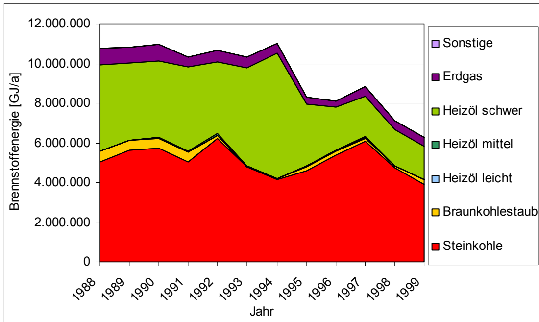
Abbildung 6: Brennstoffenergieeinsatz KET der Jahre 1988-1999 [Daten aus: HACKL & MAUSCHITZ, 1995, 1997, 2001]
