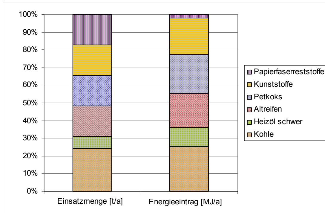
Abbildung 32: Verhältnis der Einsatzmenge und des Energieeintrags der eingesetzten Brennstoffe und Abfälle in einem fiktiven Zementwerk
