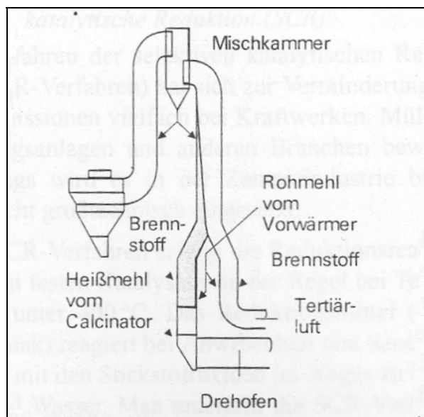
Abbildung 27: Pyroclon Low NO x Kalzinator [VDI, 2001]
