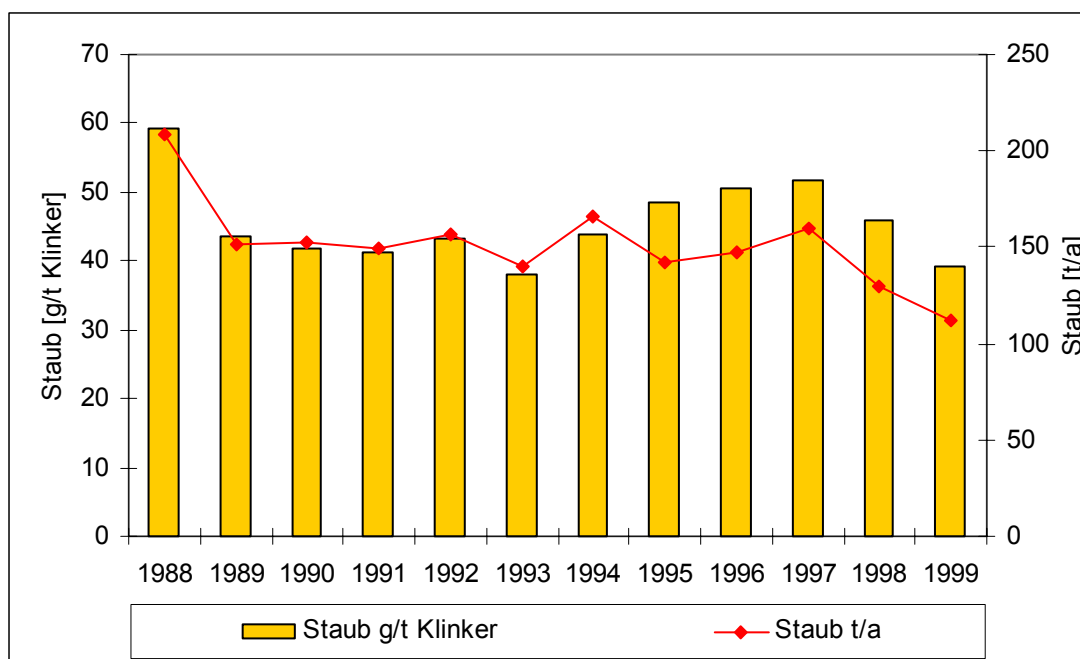
Abbildung 15: Spezifische und Gesamtstaubemissionen der österreichischen Zementindustrie 1988-1999 [Daten aus: HACKL & MAUSCHITZ, 1995, 1997, 2001]
