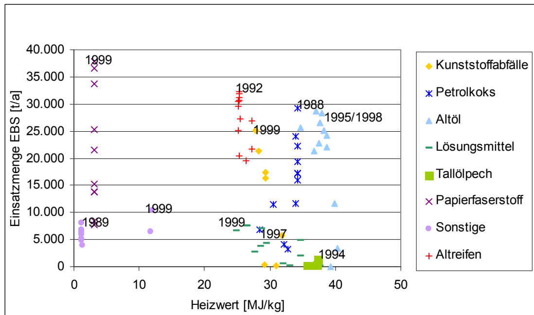
Abbildung 9: Heizwerte von Ersatzbrennstoffen und die eingesetzten Mengen der jeweiligen Brennstoffe (1988-1999). [Daten aus: HACKL & MAUSCHITZ, 1995, 1997, 2001]
