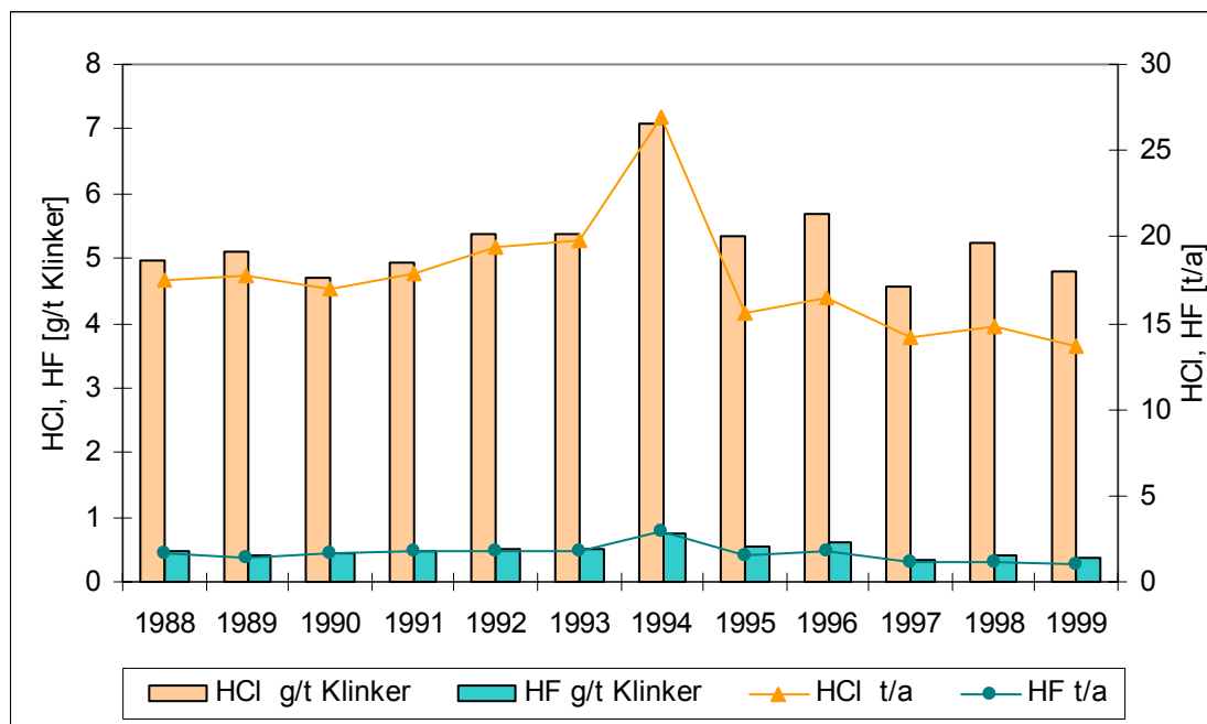
Abbildung 20: Spezifische und Gesamtemissionen von HCl und HF aus allen Zementwerken 1988-1999 [Daten aus: HACKL &amp; MAUSCHITZ, 1995, 1997, 2001]
