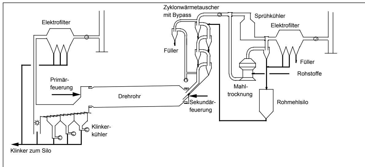
Abbildung 21: Klinkerproduktion im Trockenverfahren ohne Vorkalzinators [STUBENVOLL, 1998]
