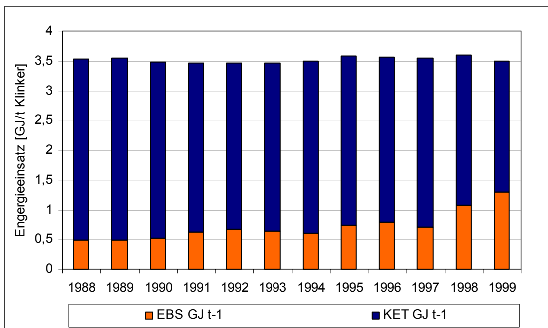
Abbildung 3: Spezifischer Energieeinsatz 1988-1999 [Daten aus: HACKL & MAUSCHITZ, 1995, 1997, 2001]
