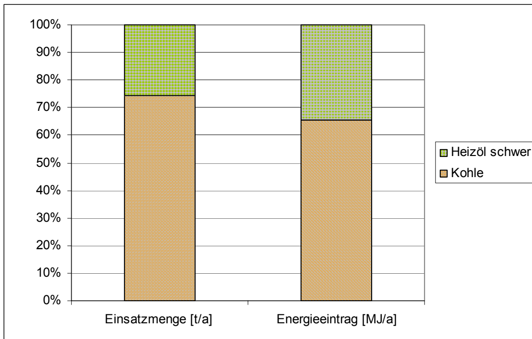
Abbildung 31: Verhältnis der Einsatzmenge und des Energieeintrags von Kohle zu Heizöl schwer in einem fiktiven Zementwerk
