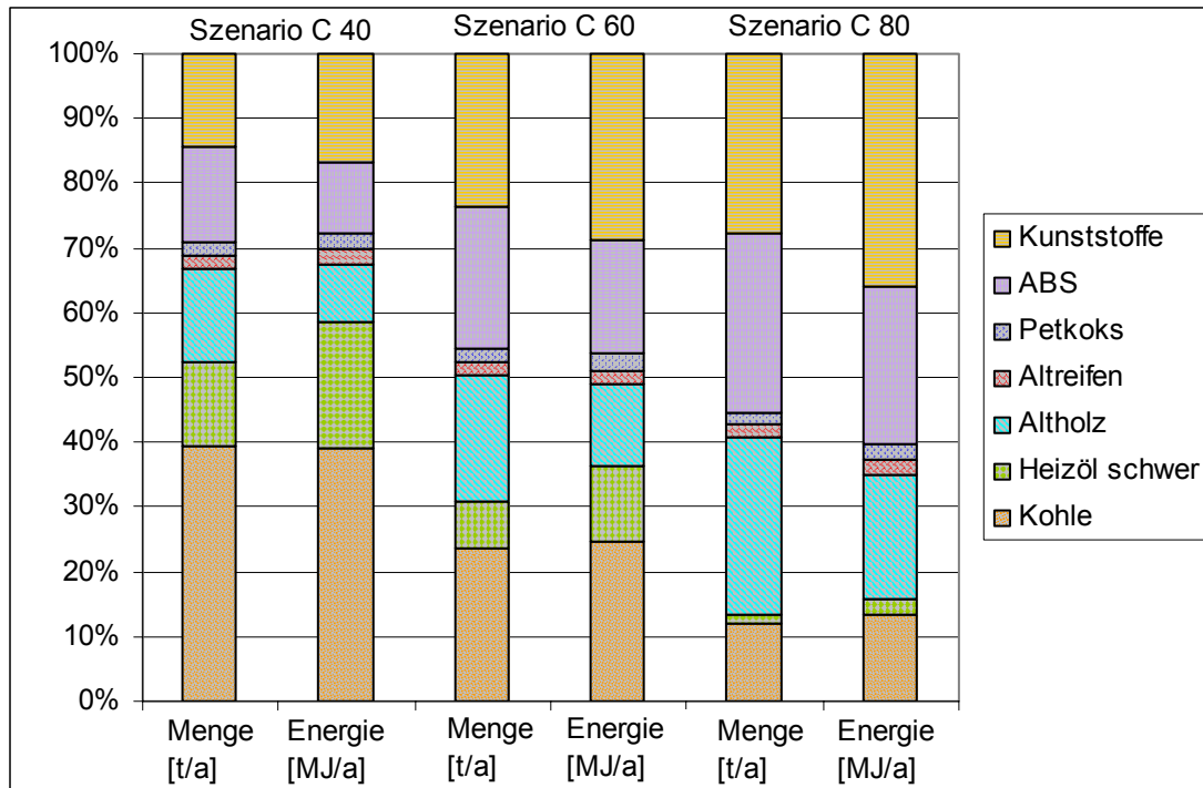
Abbildung 33: Verhältnis der Einsatzmenge und des Energieeintrags der eingesetzten Abfälle und Brennstoffe in einem fiktiven Zementwerk
