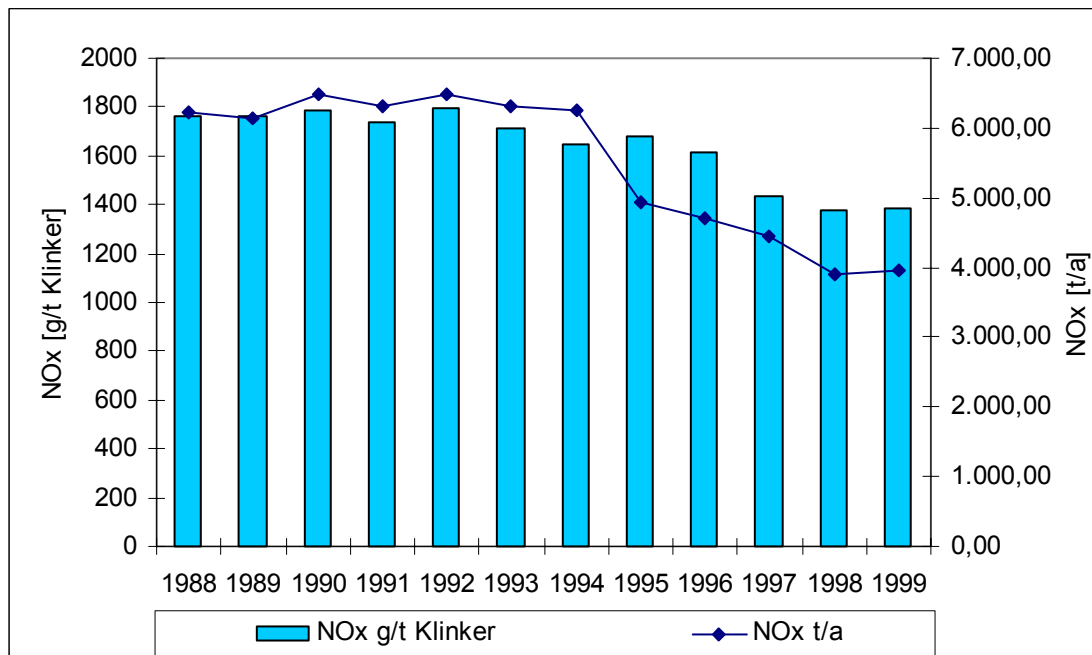
Abbildung 17: Spezifische und Gesamtemissionen von NO x der österreichischen Zementindustrie 1988-1999 [Daten aus: HACKL & MAUSCHITZ, 1995, 1997, 2001]
