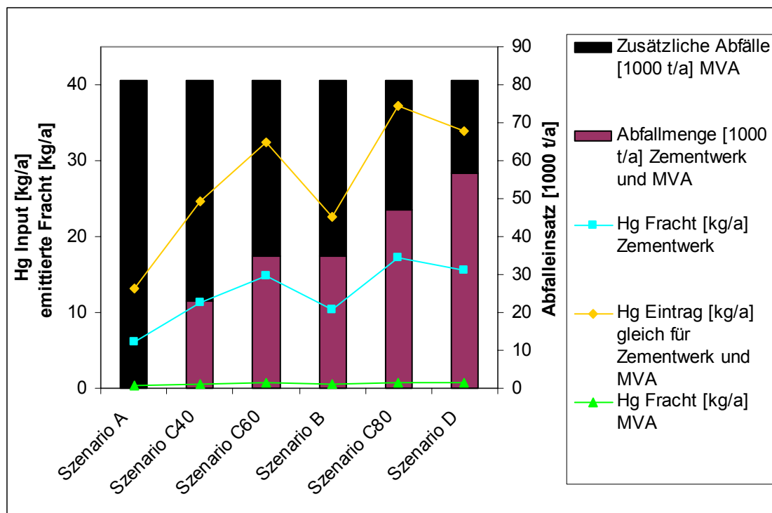
Abbildung 1: In den Szenarien A-D eingesetzte Abfallmengen und die daraus resultierenden Emissionsfrachten aus einem fiktiven Zementwert und einer Abfallverbrennungsanlage.
