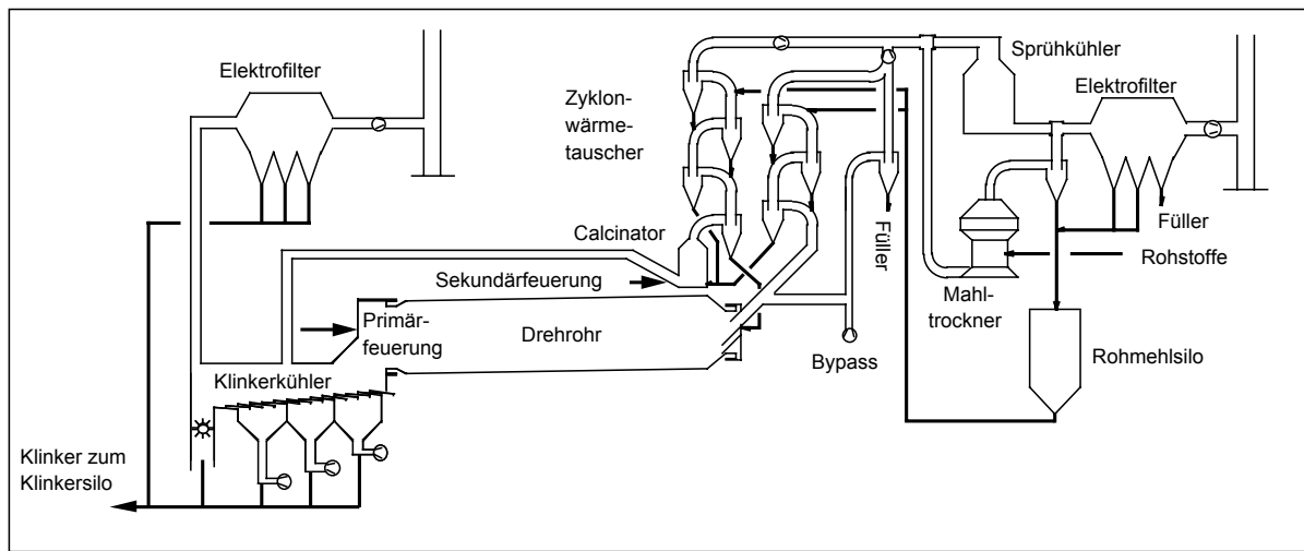
Abbildung 22: Klinkerproduktion im Trockenverfahren mit Vorkalzinator [STUBENVOLL, 1998]
