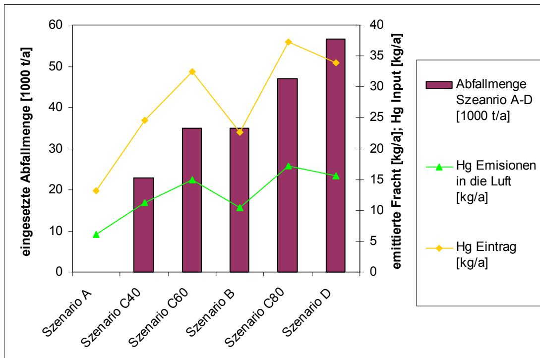
Abbildung 35: Zusammenfassung Szenario A-D des fiktiven Zementwerks
