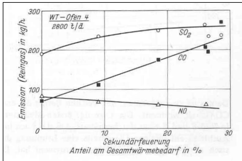
Abbildung 25: SO 2 , CO und NO Emissionen eines Zyklonvorwärmerofens mit braunkohlebefeuerter Sekundärfeuerung [SPRUNG, 1983]
