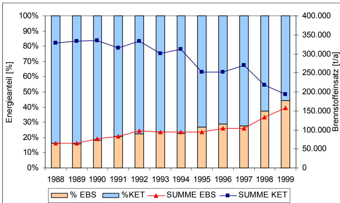
Abbildung 2: Entwicklung der konventionellen Energieträger und der Ersatzbrennstoffe von 1988-1999 [Daten aus: HACKL & MAUSCHITZ, 1995, 1997, 2001]
