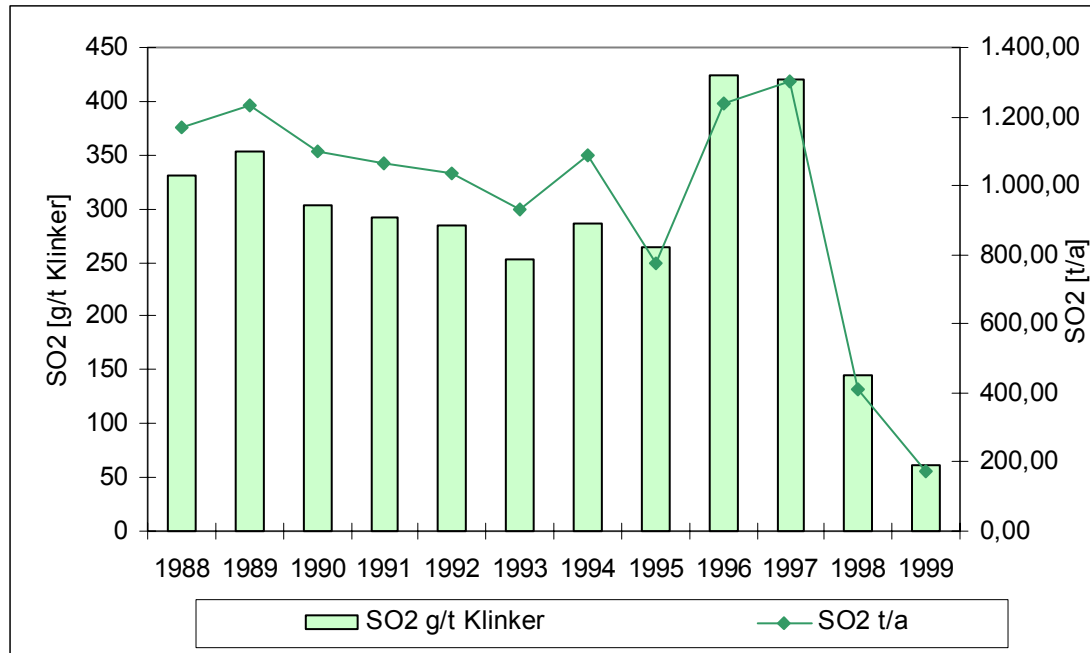
Abbildung 16: Spezifische und Gesamtemissionen von \text{SO}_2 der österreichischen Zementindustrie 1988-1999 [Daten aus: HACKL & MAUSCHITZ, 1995, 1997, 2001]
