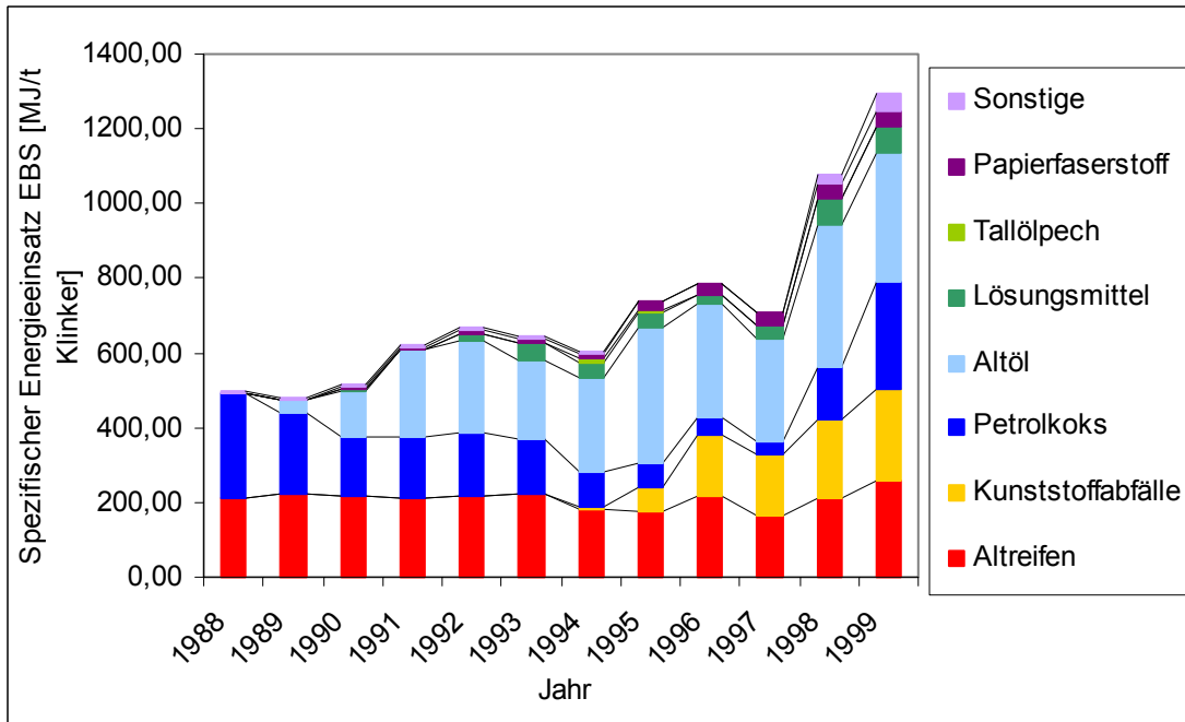
Abbildung 11: Energieeinsatz EBS der Jahre 1988-1999 bezogen auf eine Tonne Klinker [Daten aus: HACKL & MAUSCHITZ, 1995, 1997, 2001]
