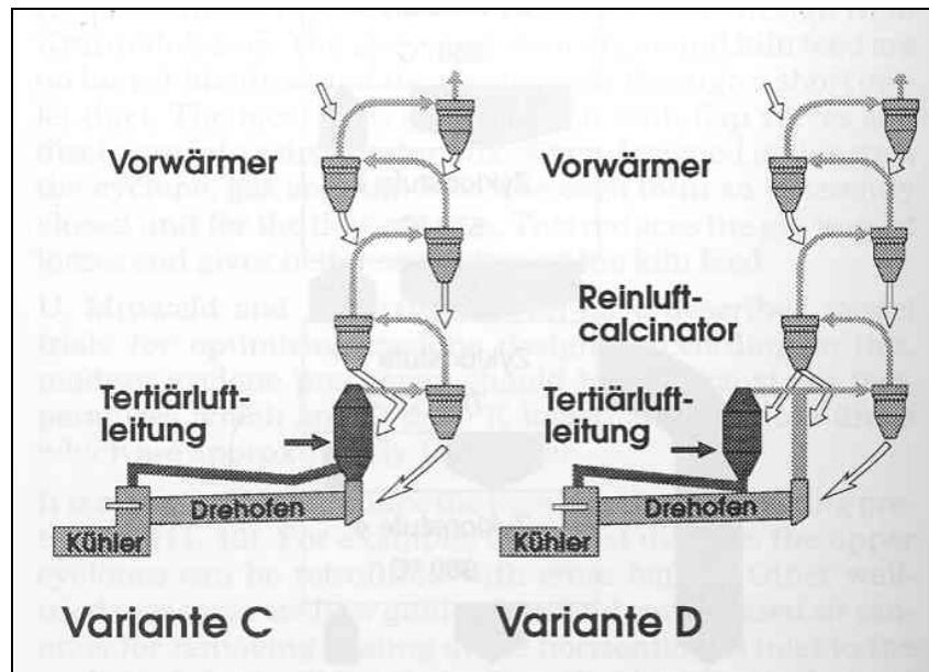
Abbildung 23: Vorkalziniervorverfahren mit Tertiärluftführung [ERHARD et al., 1994]
