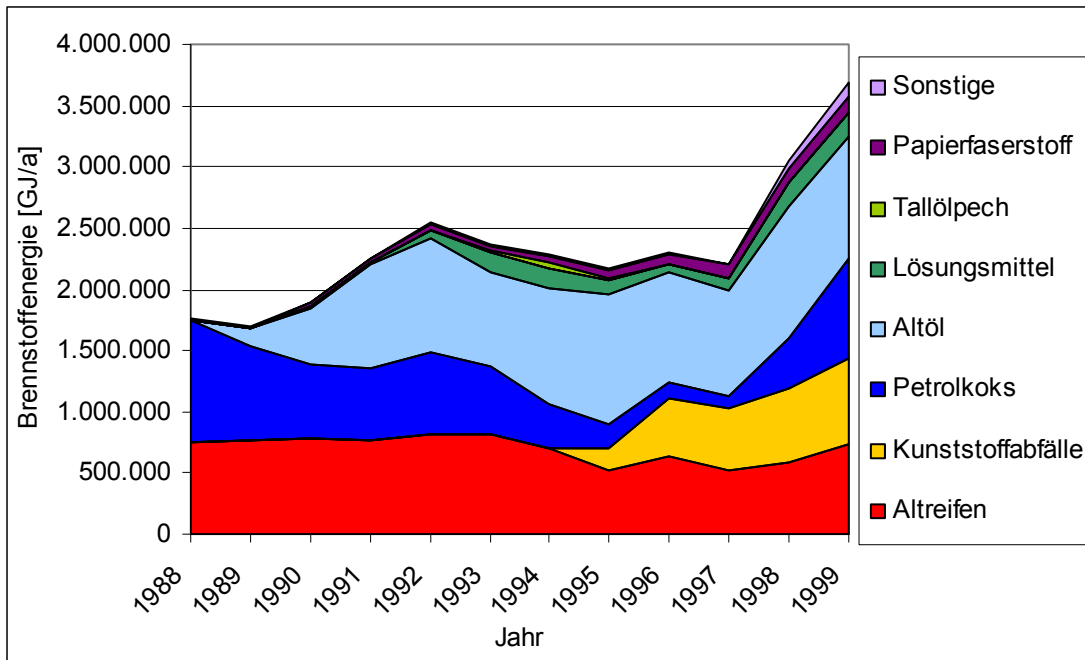
Abbildung 10: Brennstoffenergieeinsatz EBS der Jahre 1988-1999 [Daten aus: HACKL & MAUSCHITZ, 1995, 1997, 2001]
