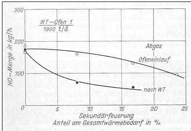
Abbildung 24: Rückgang des NO Gehalts im Ofenabgas mit zunehmendem Anteil der Sekundärfeuerung am Gesamtwärmeverbrauch eines Ofens mit Zyklonvorwärmer [SPRUNG, 1983]
