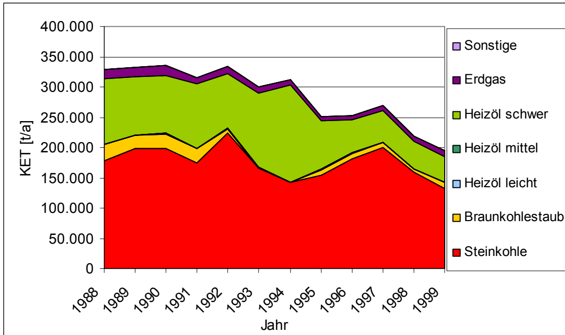
Abbildung 4: Entwicklung des Einsatzes konventioneller Brennstoffe 1988-1999 [Daten aus: HACKL & MAUSCHITZ, 1995, 1997, 2001]
