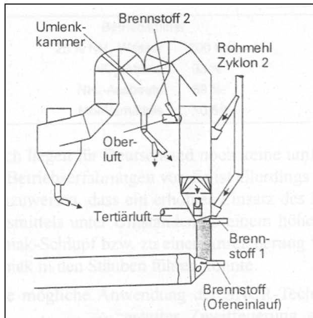
Abbildung 26: PREPOL MSC Kalzinator der Firma Krupp Polysius AG (schematische Darstellung) [VDI, 2001]
