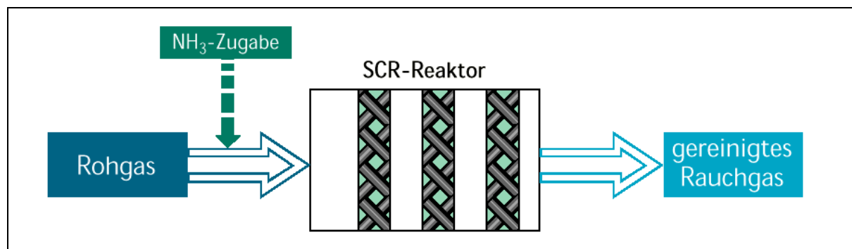
Abbildung 28: Schema des SCR-Verfahrens [VERBUNGESELLSCHAFT, 1996]
