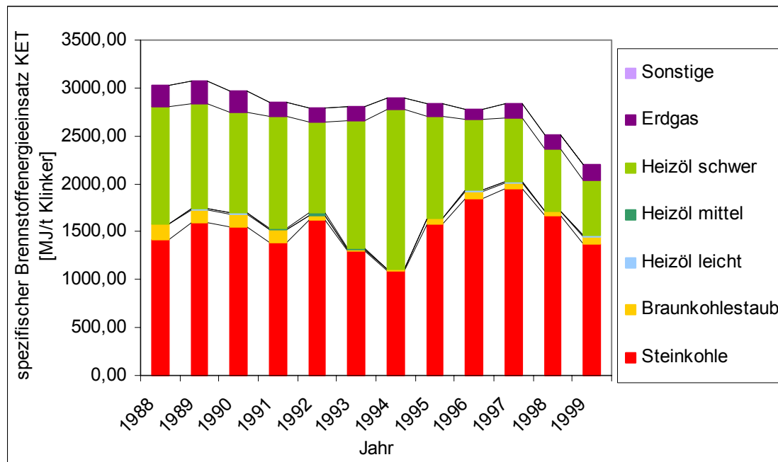
Abbildung 7: Energieeinsatz KET der Jahre 1988-1999 bezogen auf eine Tonne Klinker. [Daten aus: HACKL & MAUSCHITZ, 1995, 1997, 2001]
