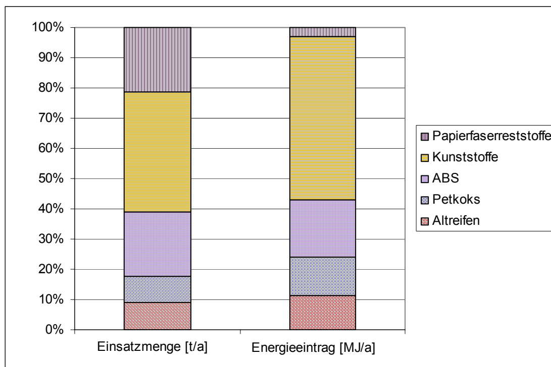
Abbildung 34: Verhältnis der Einsatzmenge und des Energieeintrags der eingesetzten Abfälle in einem fiktiven Zementwerk
