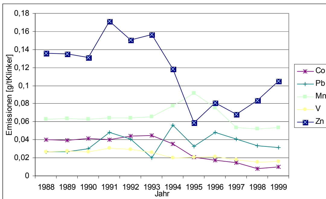
Abbildung 19: Spezifische Schwermetallemissionen 1988-1999 [Daten aus: HACKL & MAUSCHITZ, 1995, 1997, 2001]
