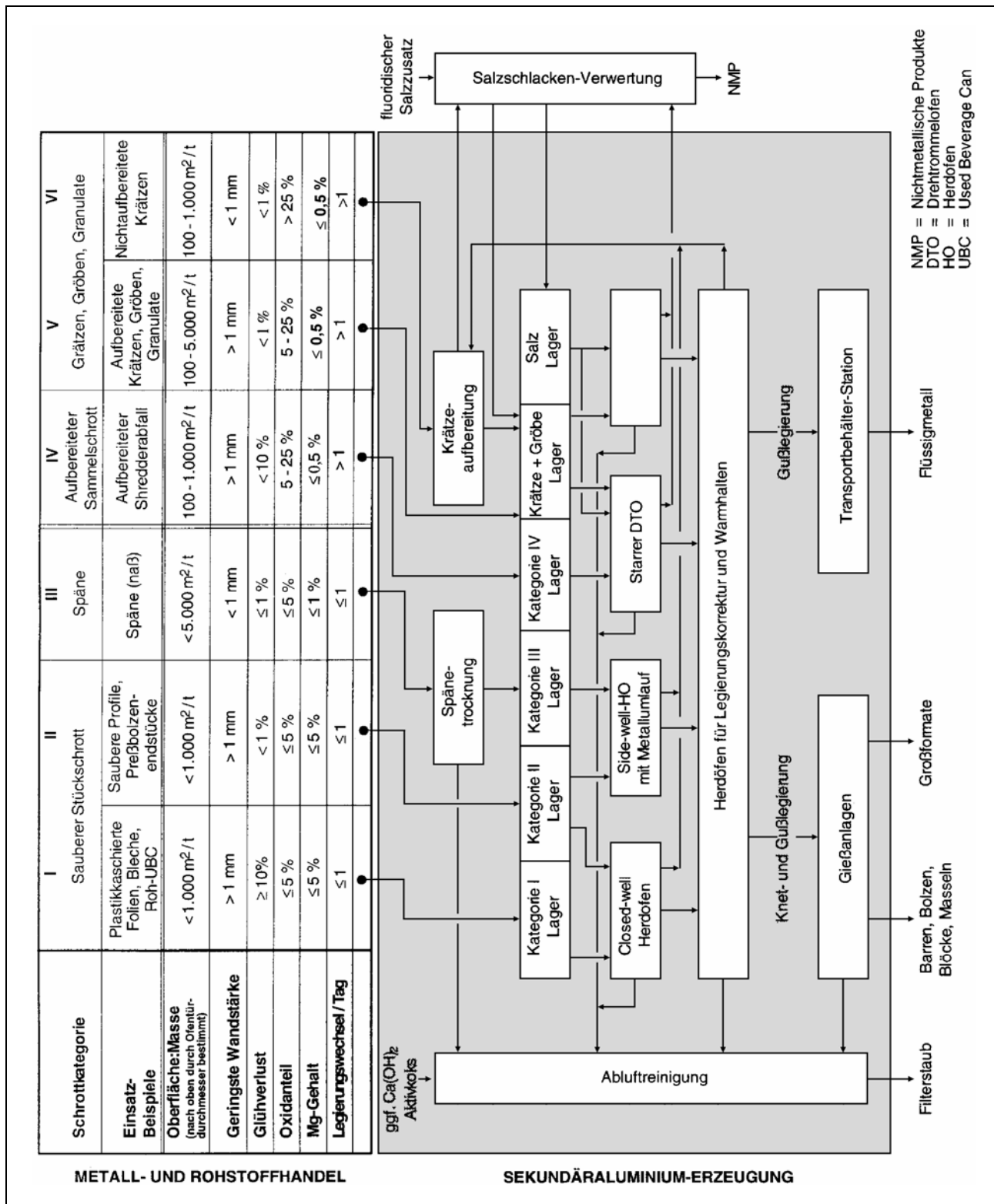
Abb. 31: Stand der Technik für die Sekundäraluminiumerzeugung zur Verarbeitung aller Schrottkategorien (UMWELTBUNDESAMT 2000).
