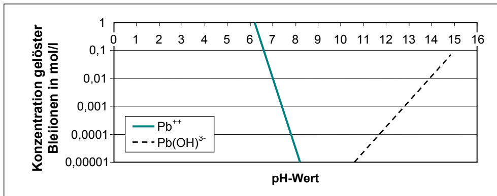
Abb. 32: Löslichkeit von Blei-Ionen als Funktion des pH-Wertes (SEEL 1973).
