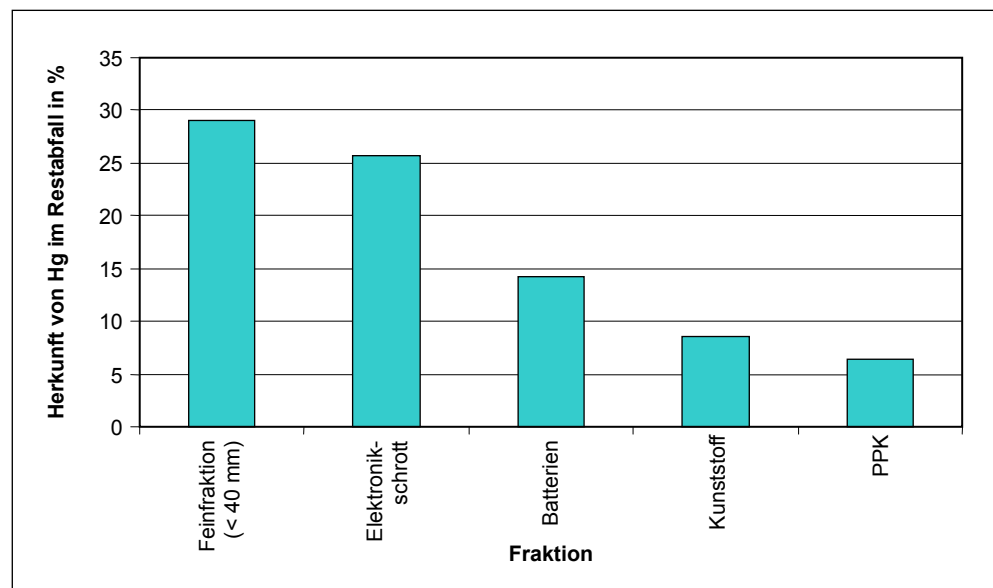
Abb. 7: Herkunft des Quecksilbers im deutschen Restabfall im Jahr 2002 (errechnet aus ROTTER 2002 und ALLGAIER & STEGMANN 2004).
