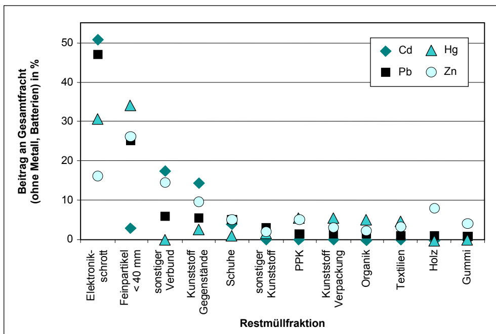
Abb. 6: Aufteilung der Gesamtfracht einzelner Schwermetalle auf die einzelnen Fraktionen sächsischen Restmülls ohne Berücksichtigung der Metall- und Batteriefractionen (ROTTER 2002) (PPK = Papier, Pappe, Karton).
