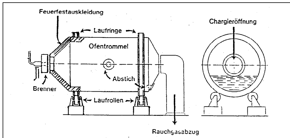
Abb. 21: Drehtrommelofen (UMWELTBUNDESAMT 2000).
