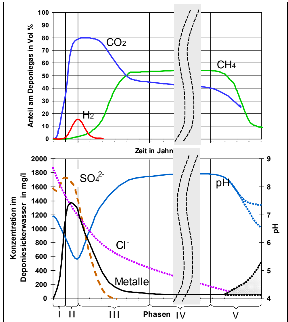
Abbildung 39: Nach Phasen des anaeroben Abbauprozesses aufgeschlüsselte Zusammensetzung von Deponiegas und -sickerwasser.
