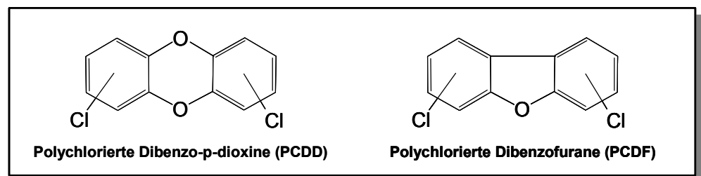
Abbildung 30: Strukturformel der Dioxine.
