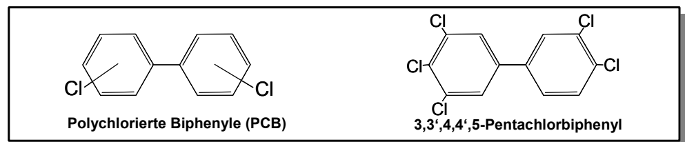
Abbildung 31: Strukturformel der polychlorierten Biphenyle (PCB).
