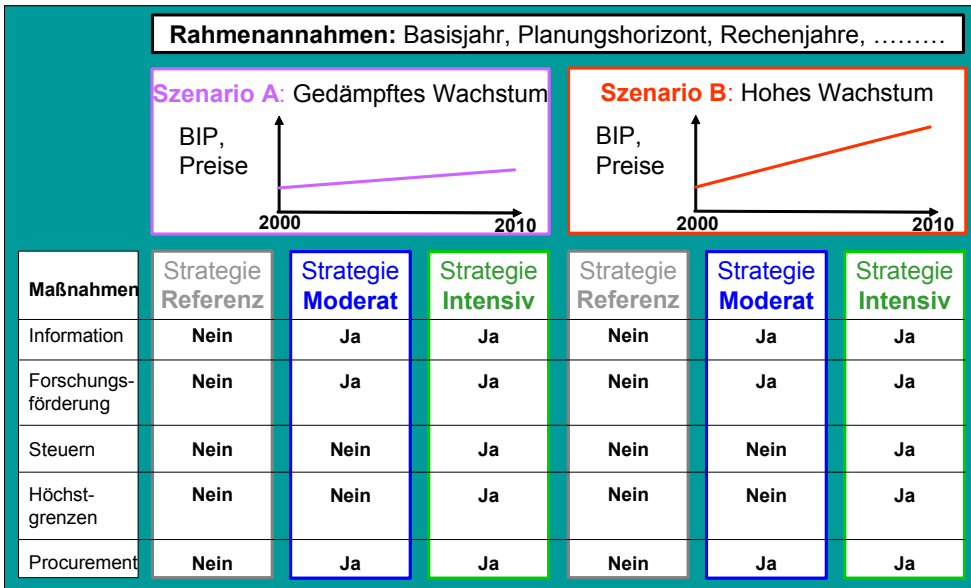
Abbildung 24: Strategie-Management-Tableau (SMT).
