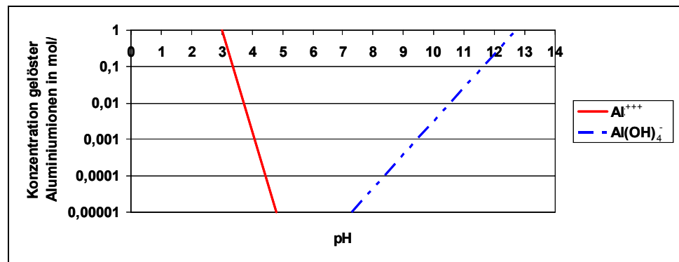
Abbildung 29: Löslichkeit von Aluminiumionen als Funktion des pH-Wertes (SEEL 1973).
