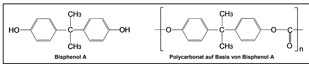
Abbildung 34: Strukturformeln von Bisphenol A und den davon abgeleiteten Polycarbonaten.
