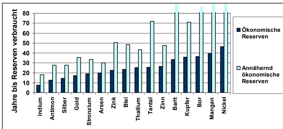
Abbildung 43: Reichweite der Metallreserven bei gegenwärtigem Ressourcenverbrauch (U.S.GEOLOGICAL SURVEY 2003).
