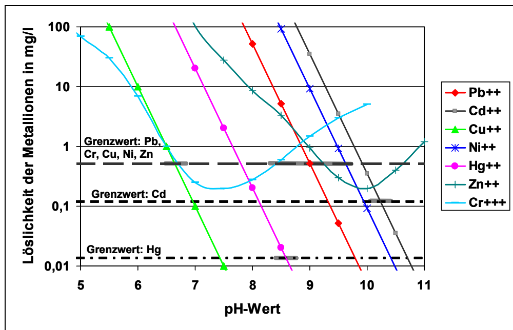
Abbildung 40: Löslichkeit von Metallionen in Abhängigkeit vom pH-Wert (WEISSENBACH 1999, SEEL 1973).
