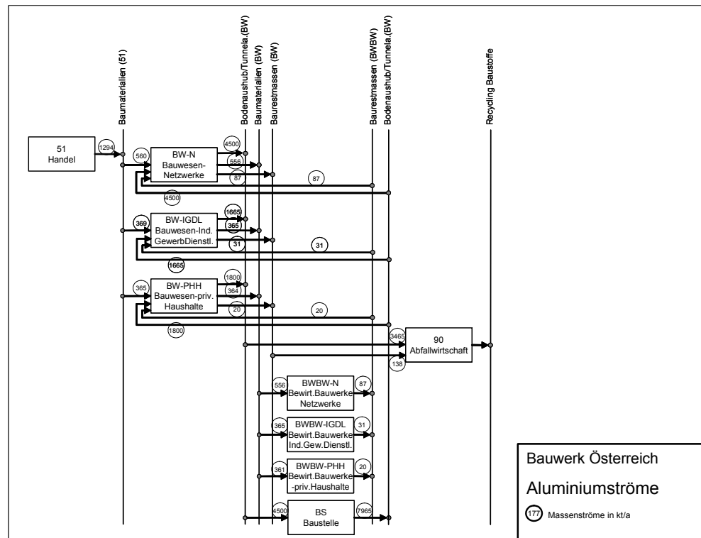
Abbildung 17: Aluminiumflüsse durch das System „Bauwerk Österreich“ für das Jahr 2001 (VOGEL-LAHNER 2003).
