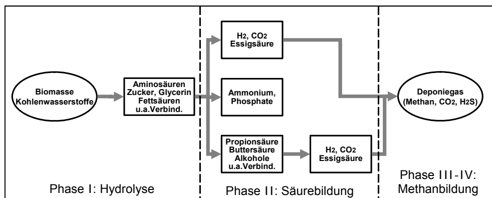
Abbildung 38: Phasen des anaeroben Abbauprozesses von Abfall in einer Hausmülldeponie.
