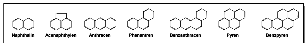
Abbildung 32: Strukturformel einiger polycyclischer aromatischer Kohlenwasserstoffe (PAK).
