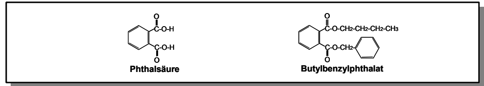
Abbildung 33: Strukturformel der Phthalsäure und eines ihrer Ester.
