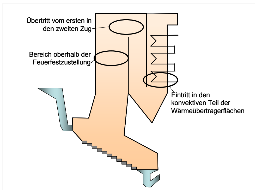
Abbildung 42: Hochtemperaturkorrosionszonen in einem Abfallverbrennungskessel (BENDIX et al.2005).
