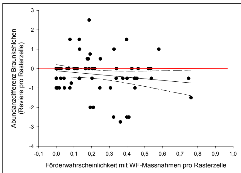
Abb. 31: Zusammenhang zwischen der Wahrscheinlichkeit des Auftretens von WF-Maßnahmen im Jahr 2003 und den Bestandsänderungen des Braunkehlchens zwischen 1998–2005 pro ornithologischer Rasterzelle á 6,25 ha. Punkte unterhalb der roten Nulllinie bezeichnen Rasterzellen mit Bestandsabnahmen, Punkte oberhalb der Nulllinie solche mit Bestandszunahmen. Ergebnis nicht signifikant.
