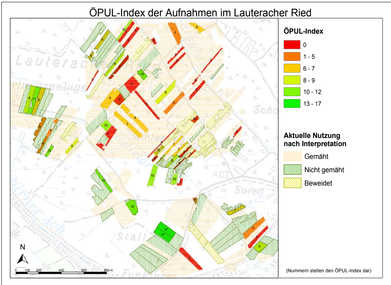
Abb. 16: ÖPUL-Index der Aufnahmen.
