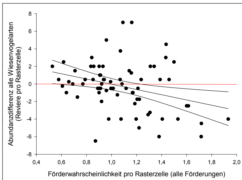
Abb. 30: Zusammenhang zwischen der Wahrscheinlichkeit des Auftretens aller ÖPUL-Maßnahmen im Jahr 2003 und den Bestandsänderungen aller Wiesenvogelarten zwischen 1998–2005 pro ornithologischer Rasterzelle á 6,25 ha. Punkte unterhalb der roten Nulllinie bezeichnen Rasterzellen mit Bestandsabnahmen, Punkte oberhalb der Nulllinie solche mit Bestandszunahmen. Ergebnis nicht signifikant.
