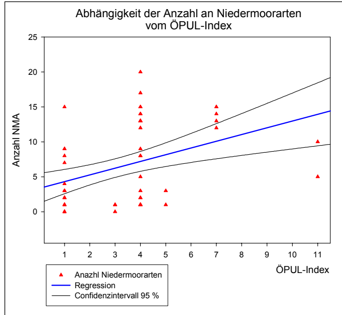
Abb. 23: Abhängigkeit der NMA-Anzahl vom ÖPUL-Index.
