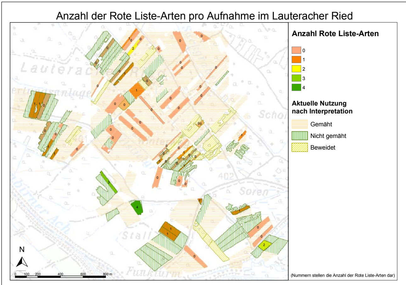
Abb. 4: Anzahl der Rote Liste-Arten.
