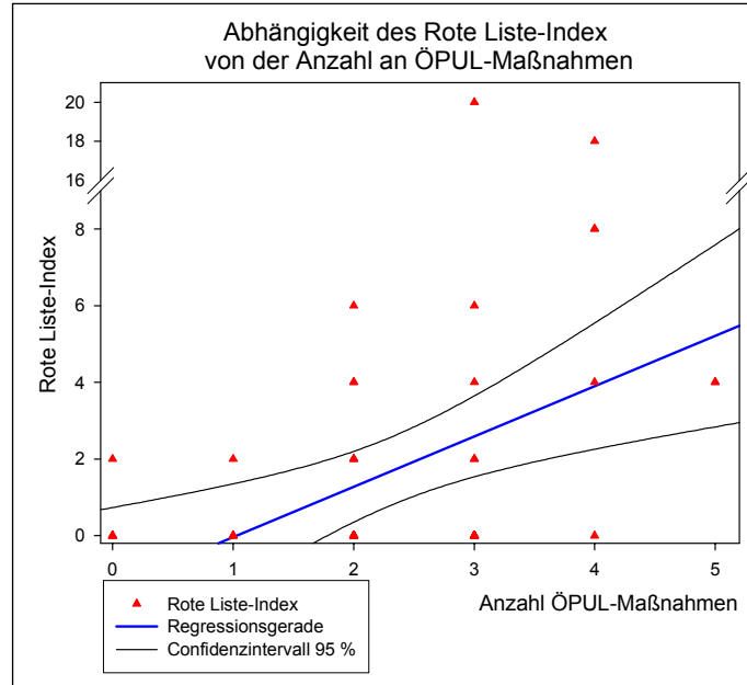
Abb. 26: Abhängigkeit des Rote Liste-Index von der Anzahl an ÖPUL-Maßnahmen.
