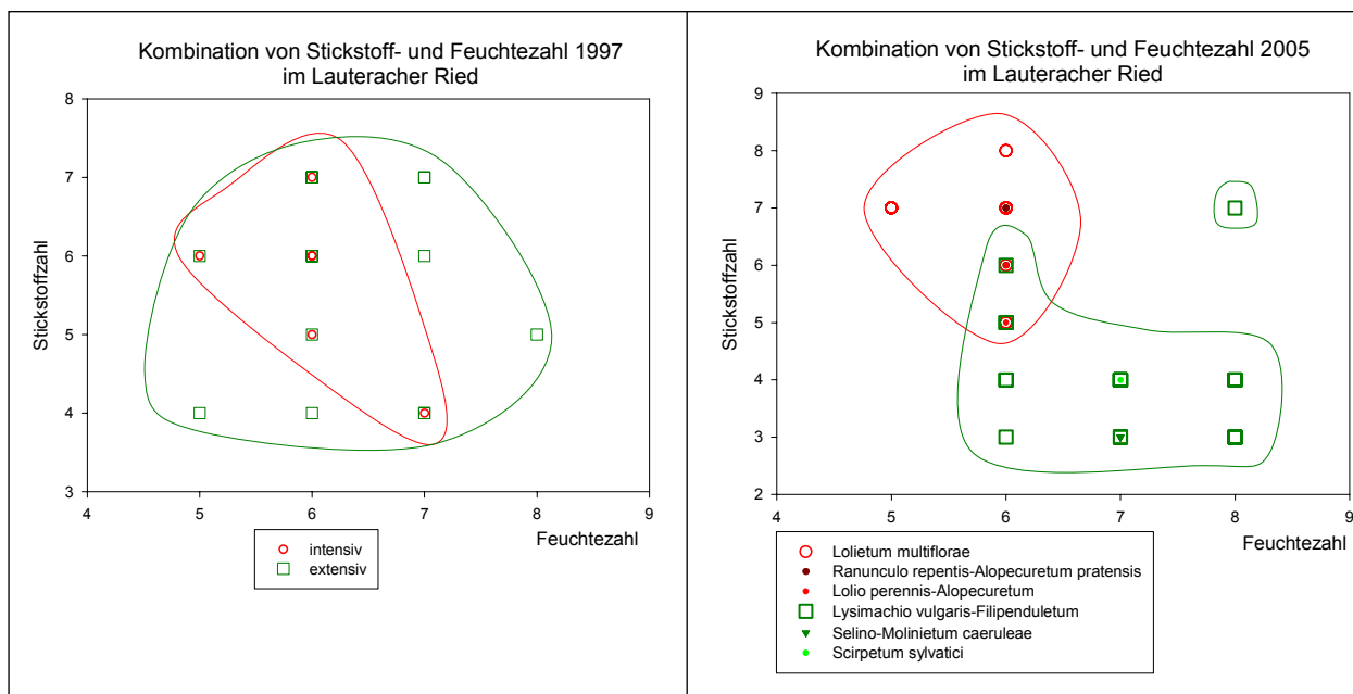
Abb. 10: Vergleich der Kombination von N- und Feuchtezahl zwischen 1997 und 2005
