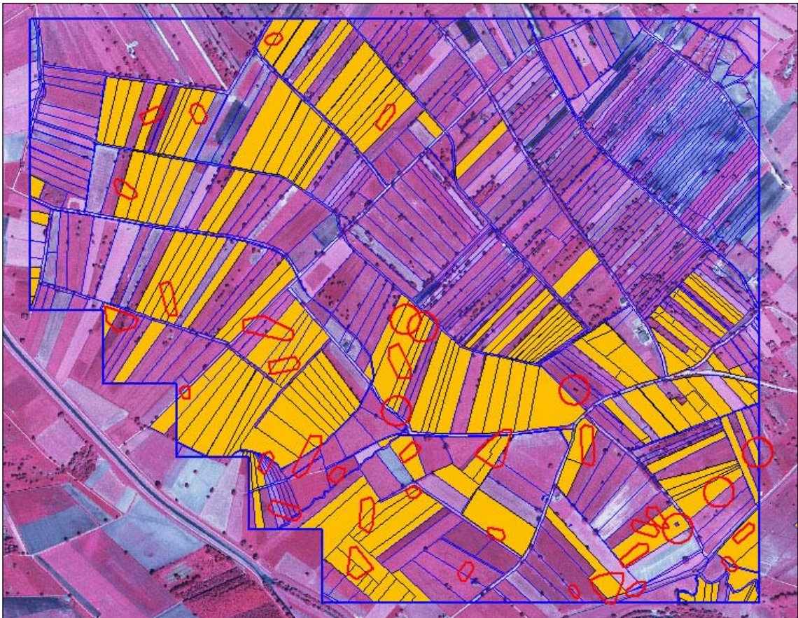
Abb. 28: Lage der Papier-Reviere des Braunkehlchens im Lauteracher Ried im Untersuchungsjahr 2005 (rote Polygone bzw. Kreise). WF-Grundstücke sind orange hervorgehoben. Braunkehlchen besiedeln statistisch signifikant häufiger WF-Grundstücke als solche ohne WF-Fördermaßnahme (Likelihood Ratio Chi-Square = 13,903, p < 0,001 ).
