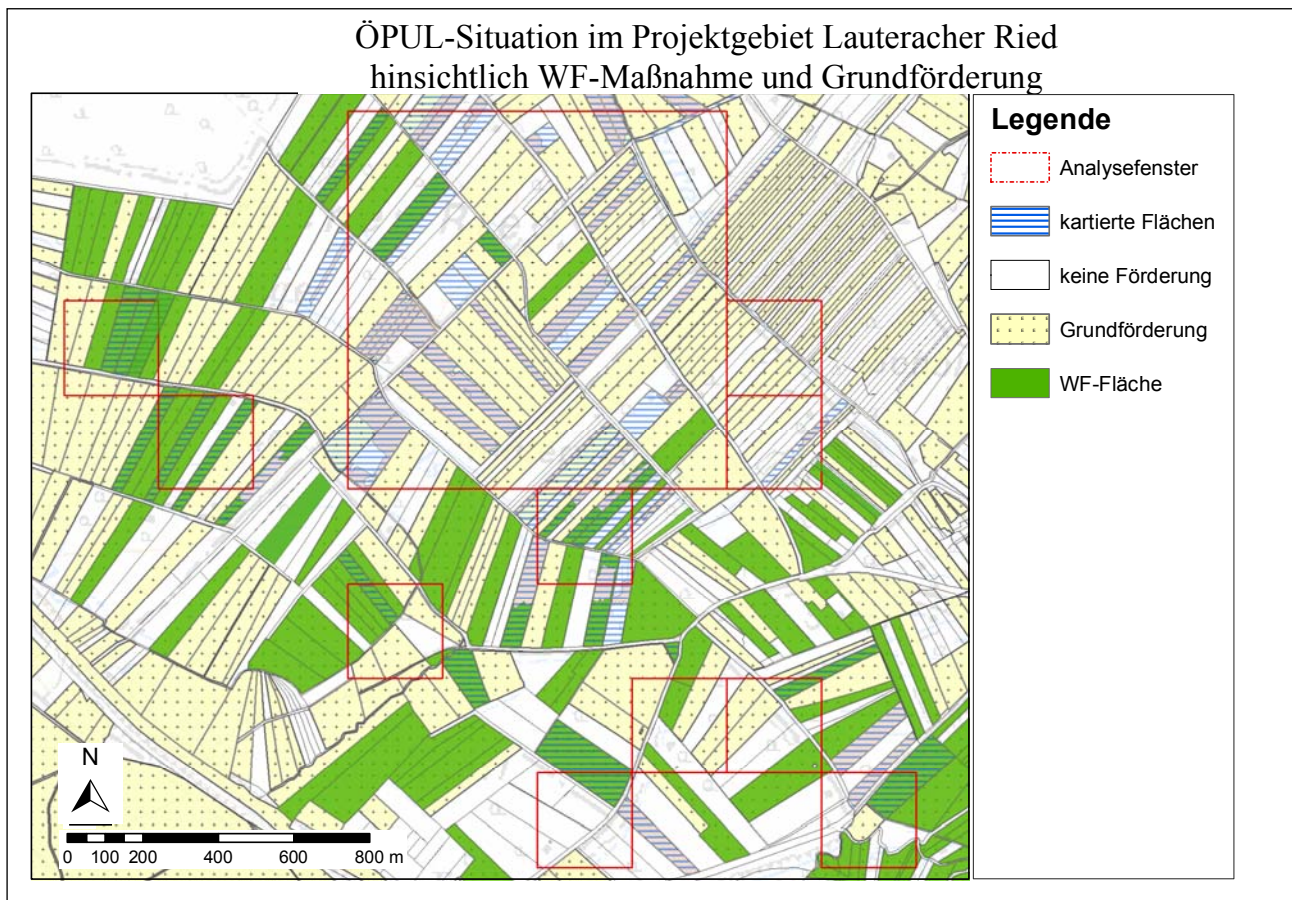
Abb. 13: ÖPUL-Situation im Lauteracher Ried.
