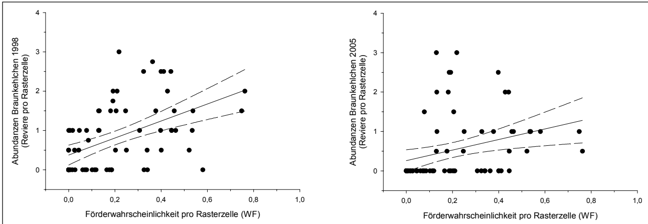
Abb. 32: Zusammenhang zwischen der Wahrscheinlichkeit des Auftretens von WF-Maßnahmen im Jahr 2003 und den Beständen des Braunkehlchens im Jahr 1998 (links; r^2 = 0,25 ) bzw. 2005 (rechts; nicht signifikant) pro ornithologischer Rasterzelle á 6,25 ha.
