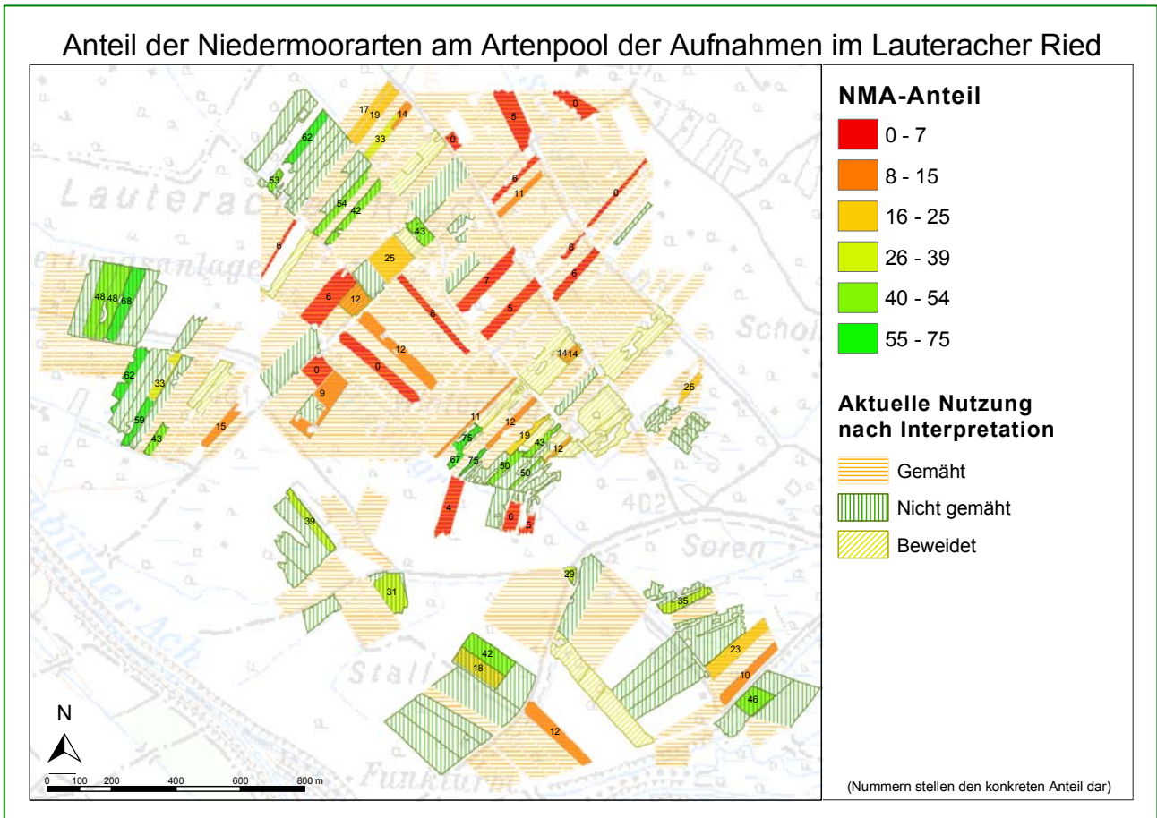
Abb. 7: Anteil der Niedermoorarten an der Gesamtartenzahl.
