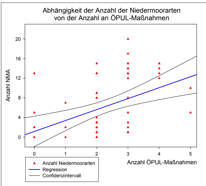
Abb. 22: Abhängigkeit der Anzahl der NMA von der Anzahl an ÖPUL-Maßnahmen.
