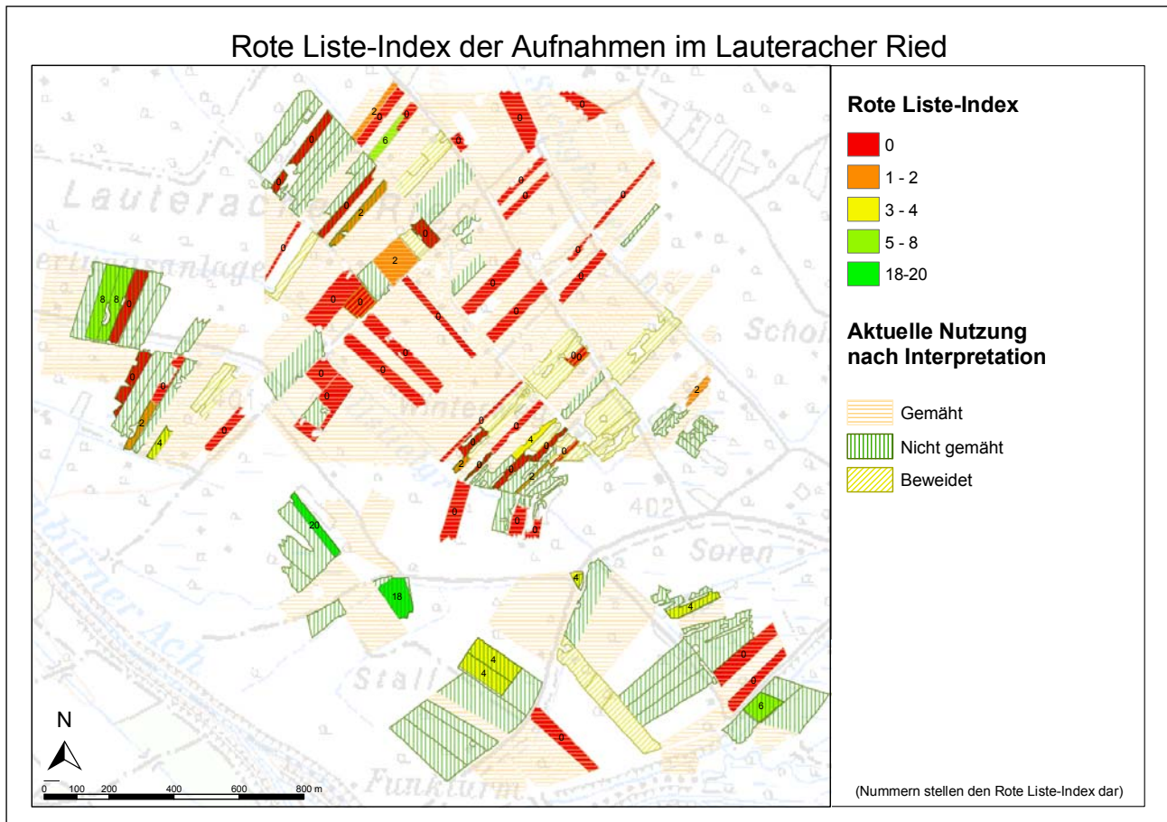
Abb. 5: Rote Liste-Index der einzelnen Aufnahmen.
