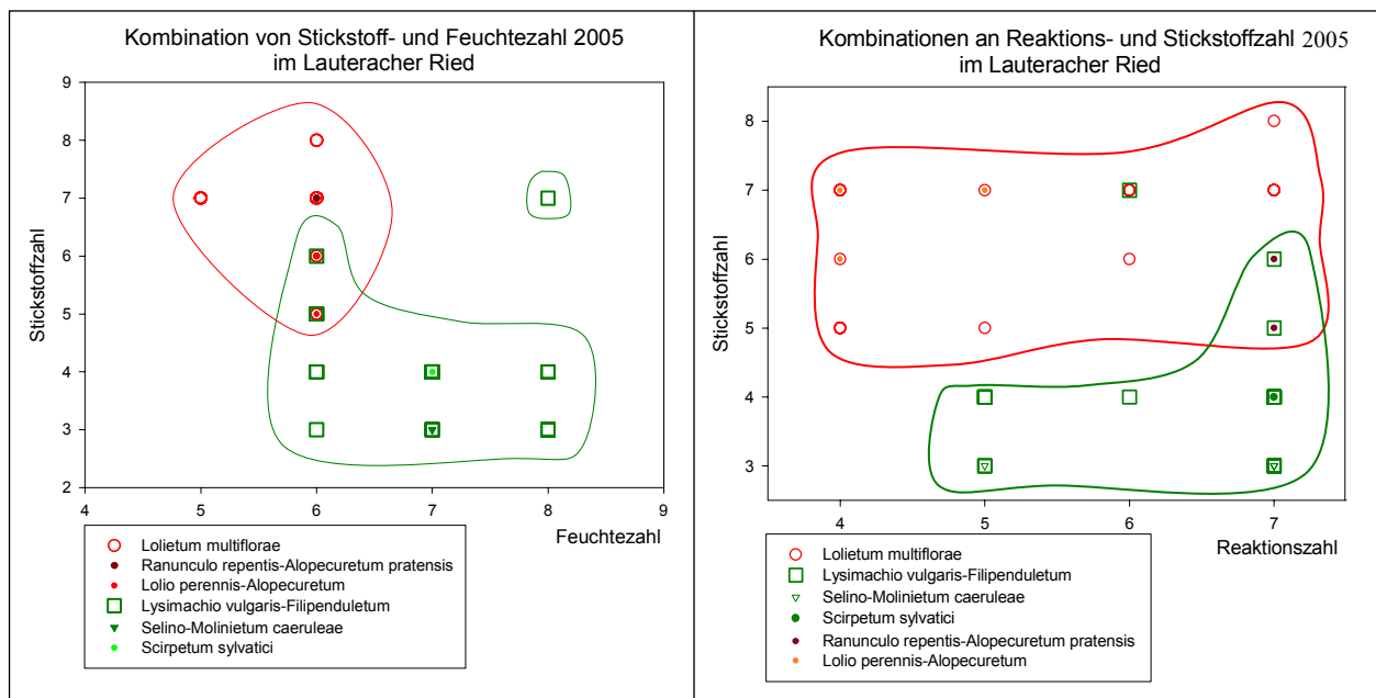
Abb. 8: Kombination von Stickstoff- und Feuchtezahl.
