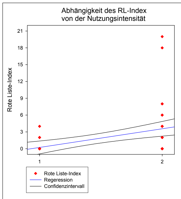
Abb. 25: Abhängigkeit des Rote Liste-Index von der Nutzungsintensität.
