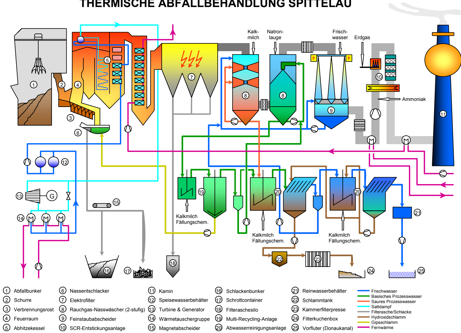
Abbildung 5: Fließbild der Müllverbrennungsanlage Spittelau.
