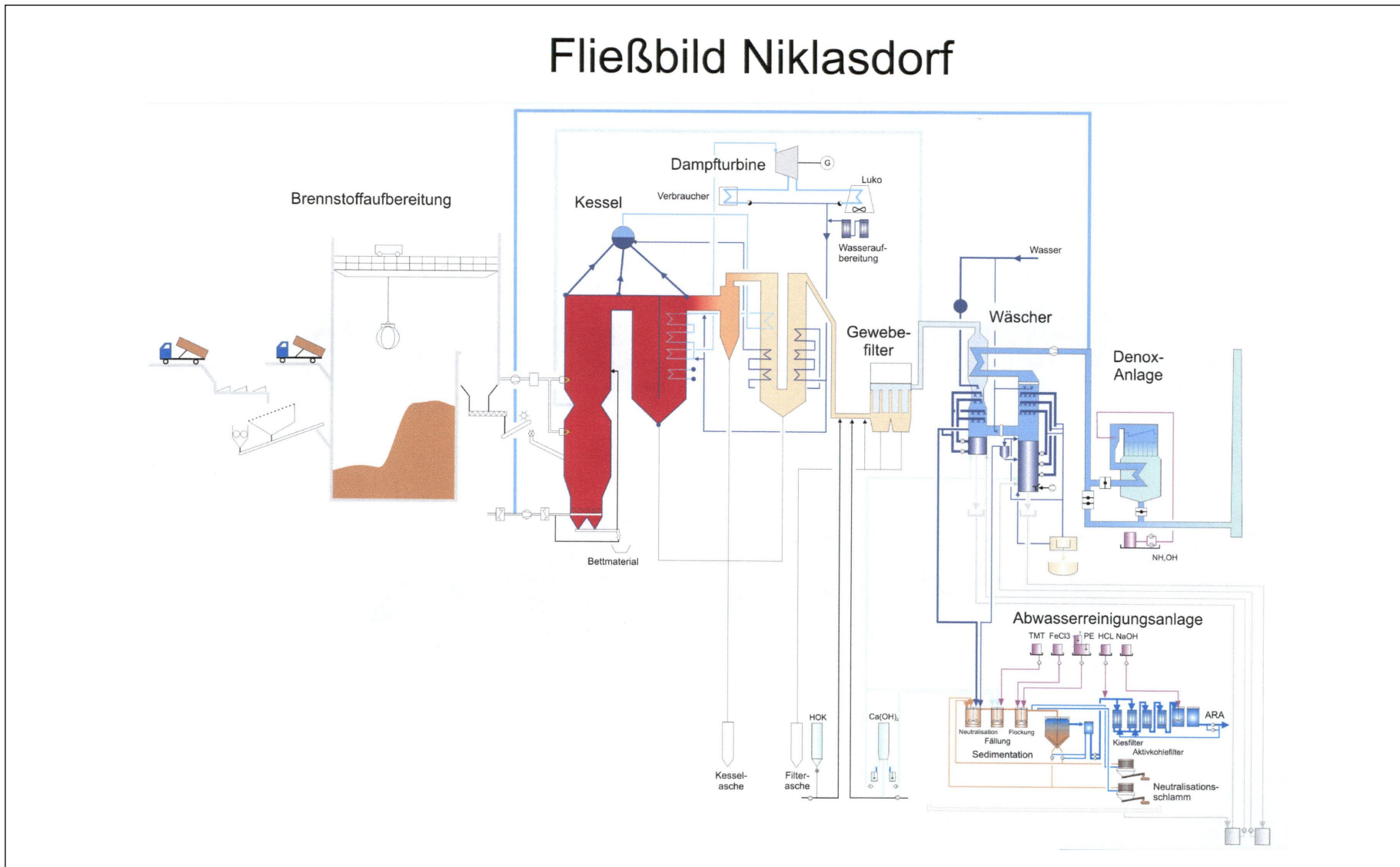
Abbildung 9: Verfahrensschema der Abfallverbrennungsanlage Niklasdorf.
