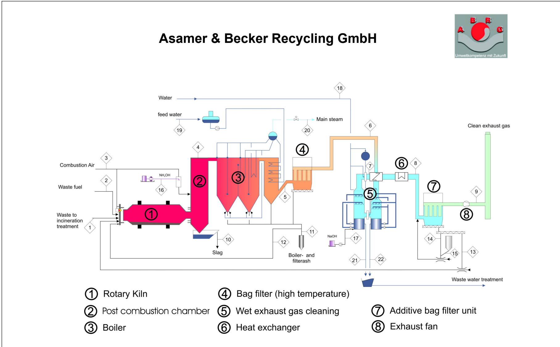
Abbildung 11: Verfahrensschema der Abfallverbrennungsanlage ABRG Arnoldstein (Drehrohrofen).
