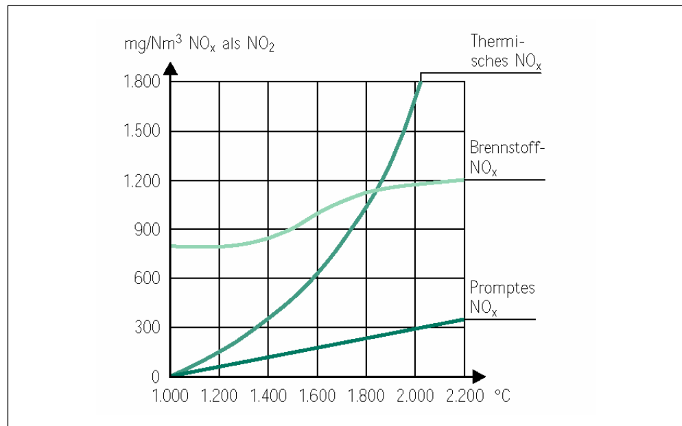
Abbildung 1: Temperaturabhängigkeit der NO x -Bildung (Umweltbericht der Verbundgesellschaft 1996, zitiert in UMWELTBUNDESAMT & TBU 2002).
