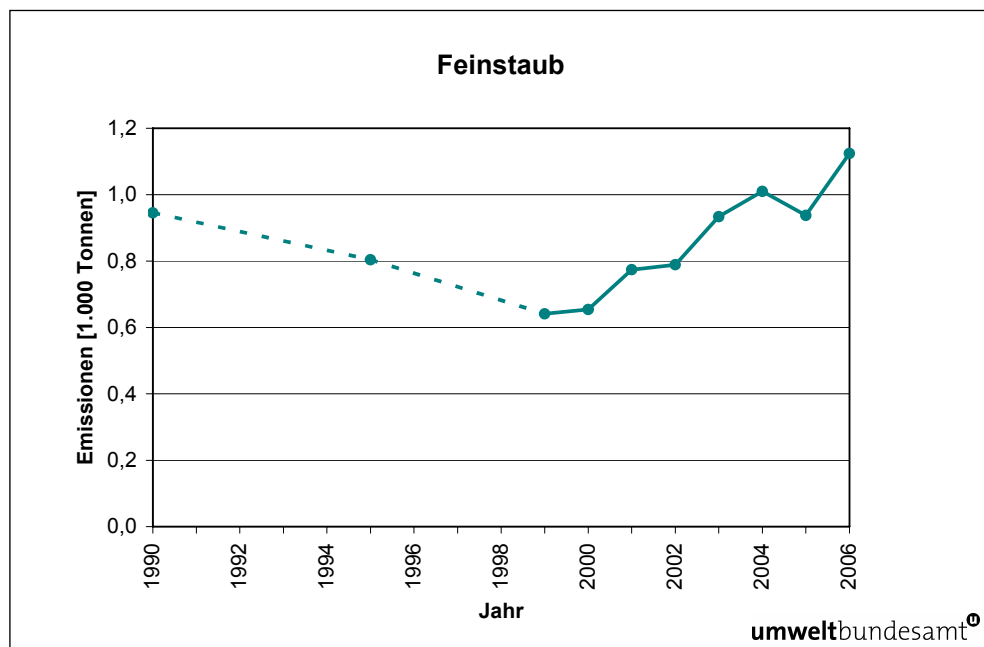
Abbildung 46: \text{PM}_{2,5} -Emissionstrend des Sektors Energieversorgung 1990–2006.
