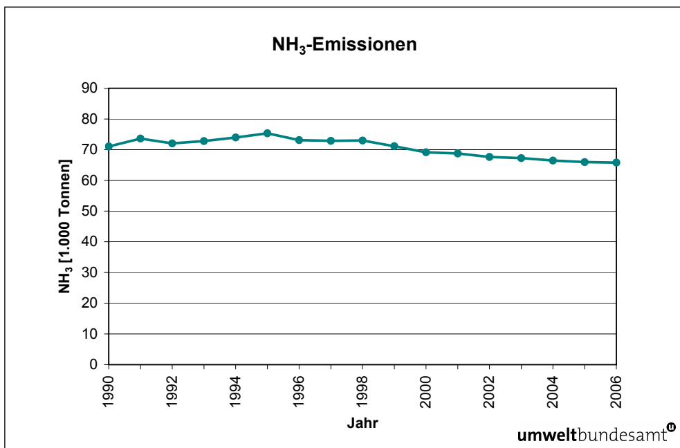
Abbildung 20: NH 3 -Emissionstrend 1990–2006.
