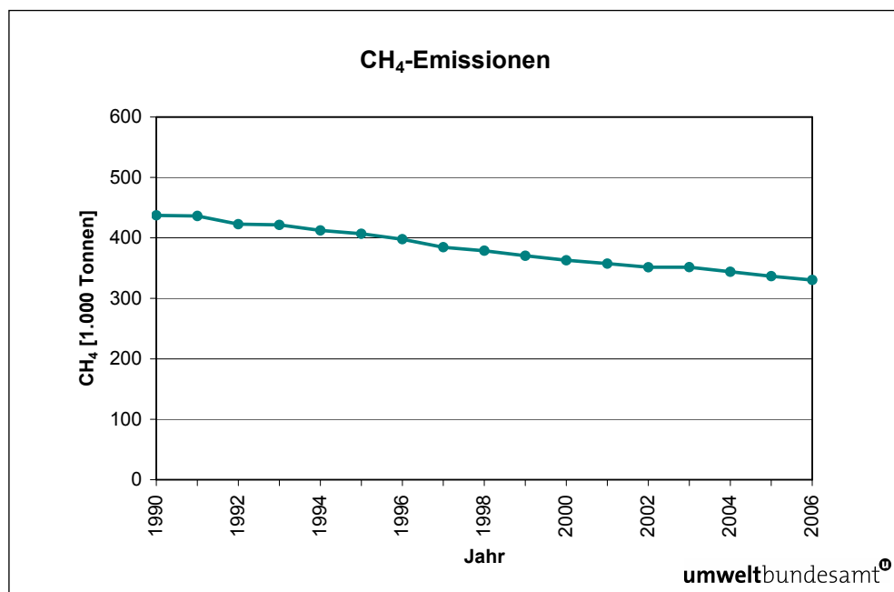
Abbildung 38: CH 4 -Emissionstrend 1990–2006.
