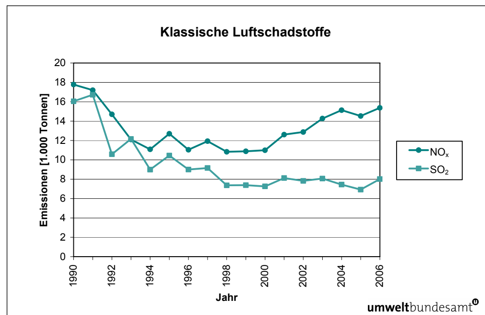
Abbildung 45: \text{NO}_x und \text{SO}_2 - Emissionstrends des Sektors Energieversorgung 1990–2006.
