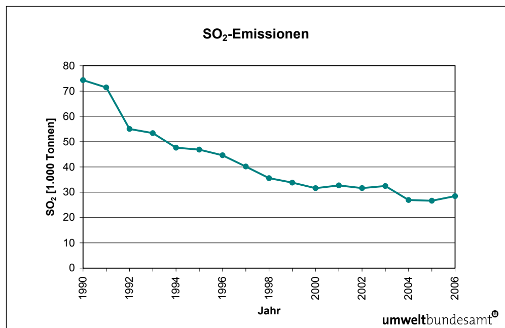
Abbildung 17: \text{SO}_2 -Emissionstrend 1990–2006.
