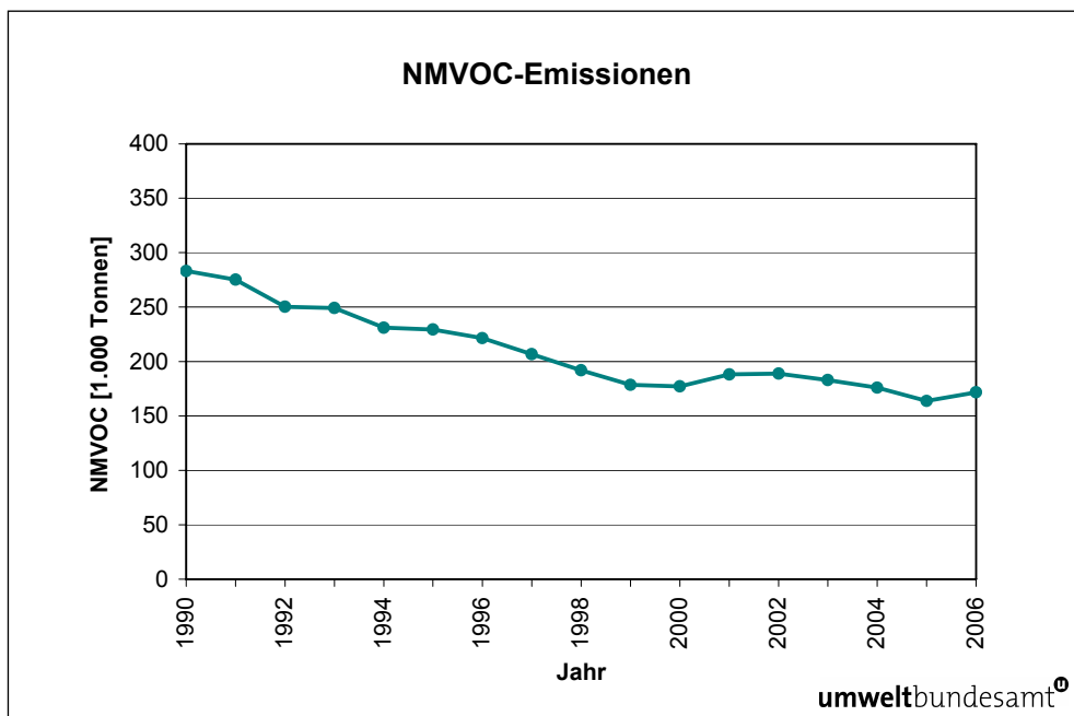
Abbildung 10: NMVOC-Emissionstrend 1990–2006.
