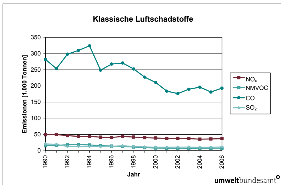
Abbildung 53: Trend der \text{NO}_x -, NMVOC-, CO- und \text{SO}_2 -Emissionen des Sektors Industrie 1990–2006.
