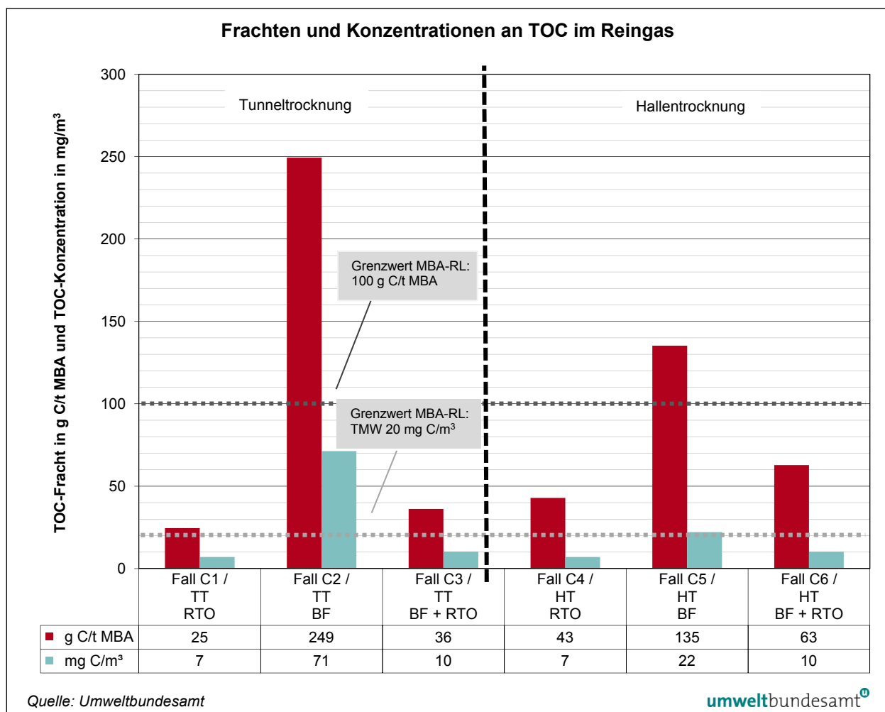
Abbildung 6: Frachten und Konzentrationen an TOC im Reingas der Anwendungsfälle C.
