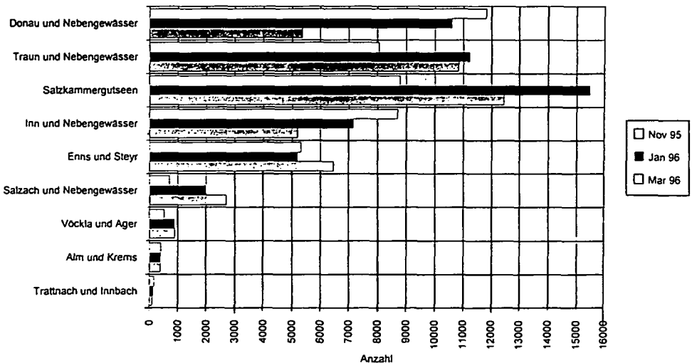
Abb. 1: Verteilung der Wasservögel in Oberösterreich auf die wichtigsten Flußeinzugsgebiete im Winter 1995/96 (November, Jänner, März).
