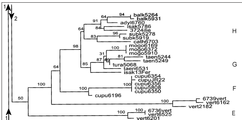
Fig. 2: Upper basal sector of a RAXML dendrogram based on ITS sequences of subg. Melanocrommyum showing the core clade at positions E - H. Numbered arrowheads mark the connections to Figs. 1 & 3. – Abb. 2: Zweiter Abschnitt eines RAXML-Dendrogramms der ITS-Sequenzen von subg. Melanocrommyum , der die Clades an den Positionen E - H zeigt. Die Pfeile und Nummern markieren die Anschlüsse zu den Abb. 1 und 3.
