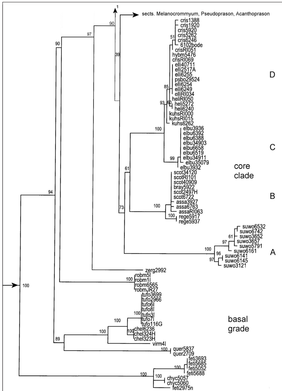
Fig. 1: Basal sector of a RAxML dendrogram based on ITS sequences of subg. Melanocrommyum showing the basal grade and the basal part of the core clade. Arrowhead 1 marks the connection to the bottom of Fig. 2. – Abb. 1: Basaler (erster) Abschnitt eines RAxML-Dendrogramms der ITS-Sequenzen von subg. Melanocrommyum , der die basalen sukzessiv abzweigenden Linien und den untersten Teil des Haupt-Clades zeigt. Pfeil 1 markiert den Anschluss zur Basis von Abb. 2.
