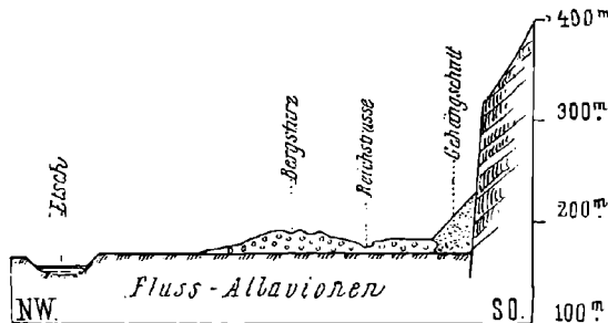
Profil über den Bergsturz südlich von S. Marco.
