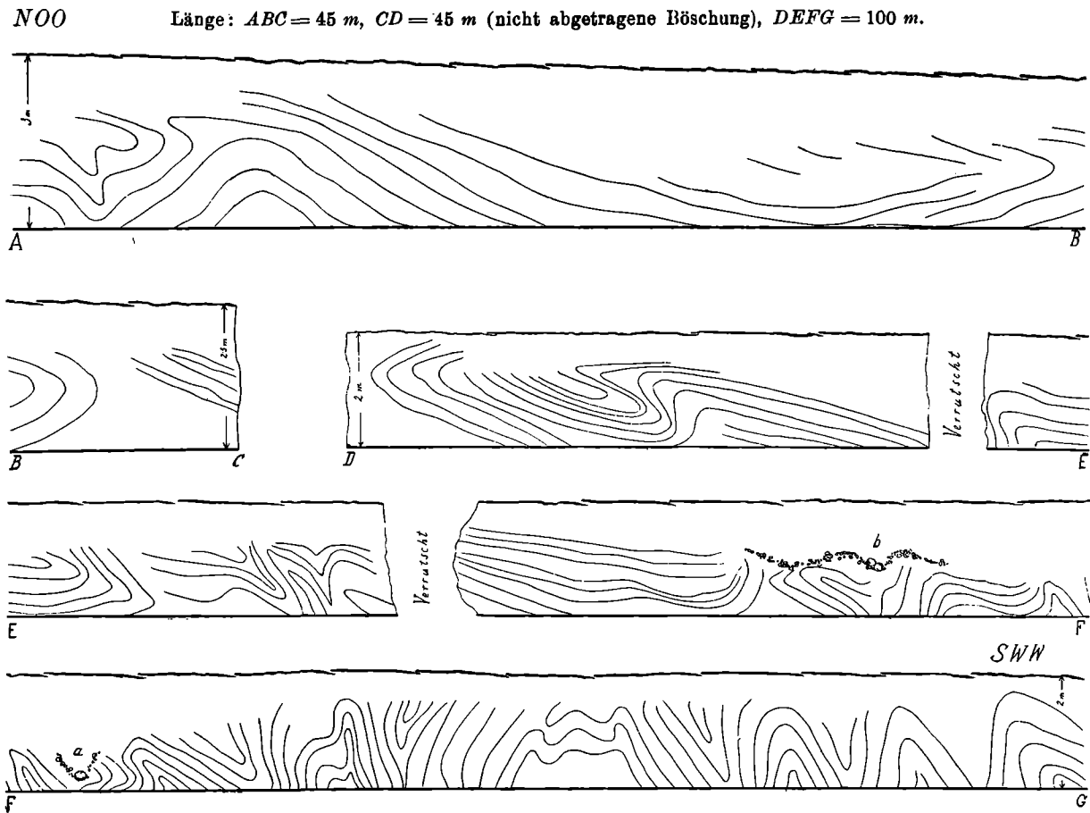
Fig. 1. Faltungen im Miocänton bei der Bahnstation Mosciska.
