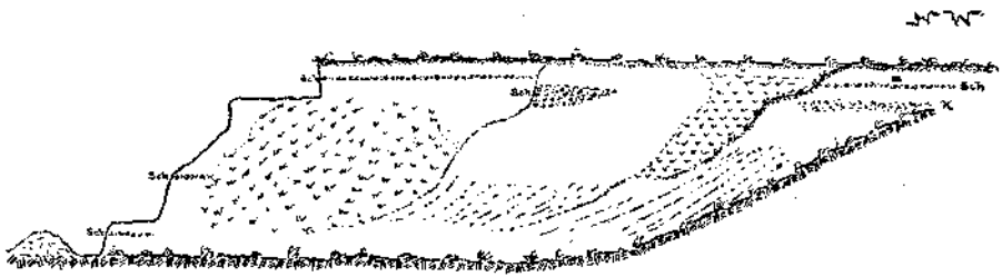
Fig. 1. Profil der Abbauwand in der östlichen Ecke des Ziegelwerkes Kraxner und Bald in St. Peter bei Graz. Sch = Schotter und Kies, K = Schicht mit Holzkohle.
