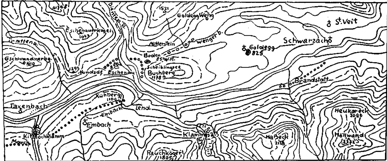
Fig. 3. Die alten Talfurchen in der Taxenbacher Enge. o-o-o-o-o pliozän? ●●●●● präglazial ooooooooo M-R Interglazial ..... R-W Interglazial Maßstab 1: 100.000
