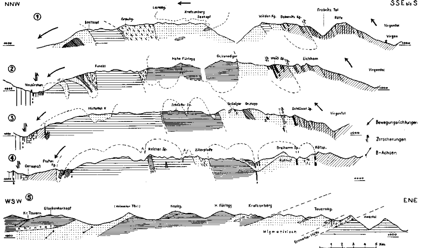
Abb. 1. Profile durch die Venediger-Gruppe. Signaturen wie auf Tafel 1
