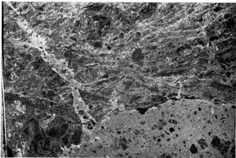
Ungestörter Intrusivkontakt von Quarzdioritporphyrit mit Mylonit der Donaustörung. Dünnschliff in Dunkelfeldbeleuchtung, ca. 3,5fach vergrößert. (Photo THIELE.)
