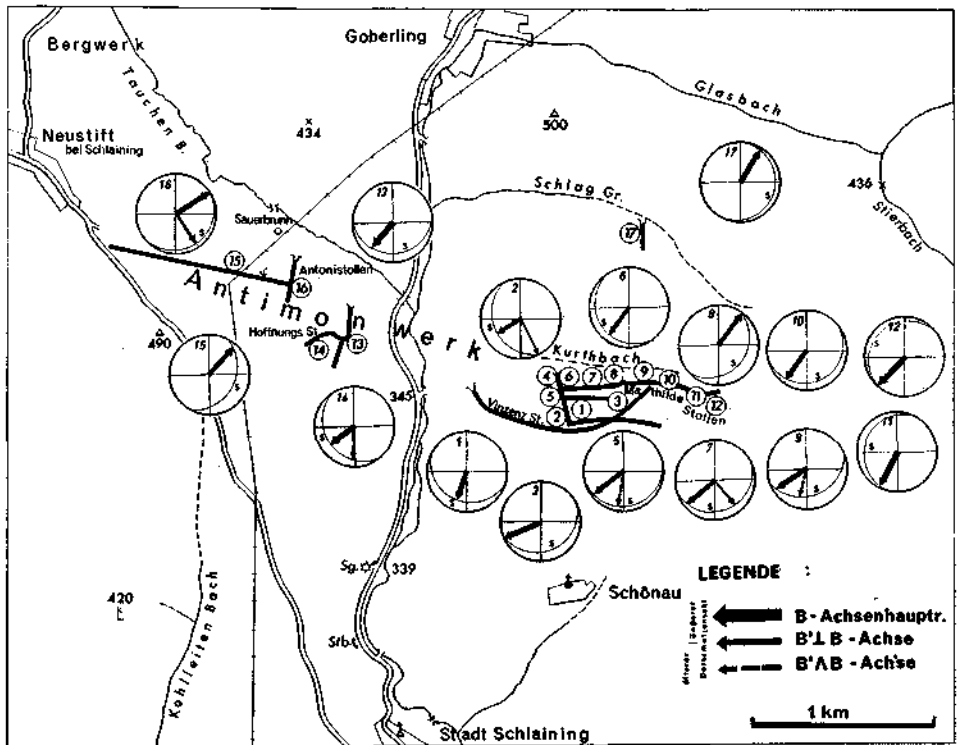
Abb. 2. Tektonische Übersichtskarte
