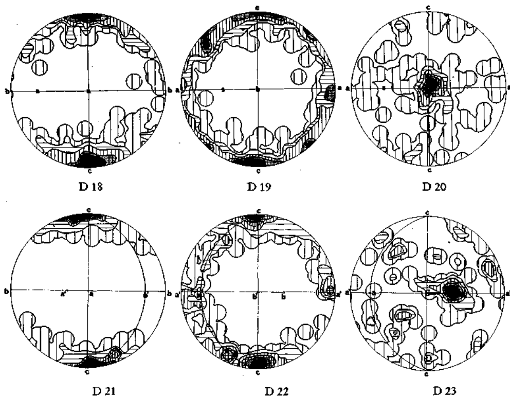
Abb. 9. Untersuchung im Mikrobereich e-Calcitlamellen (0112) und Quarzachsen
