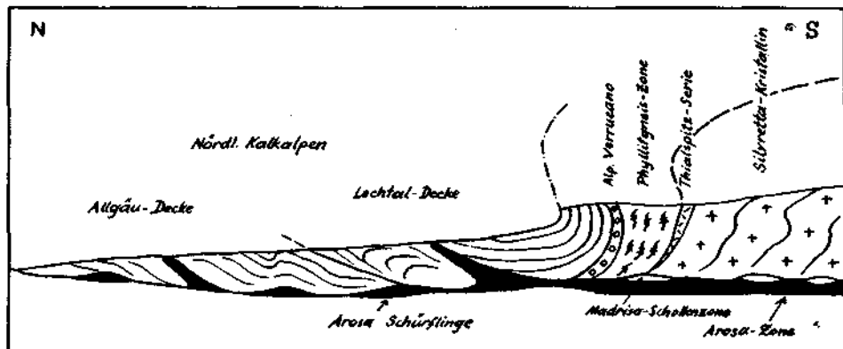
Abb. 1. Schematisches Sammelprofil der Verhältnisse nahe dem Westrand der Kalkalpen. Es soll in stark generalisierter Weise das Ausheben der Kalkalpen über dem Kristallin der Zentralalpen und die auf der einstigen Schubbahn liegenden, sekundär eingewickelten kalkalpinen Schollen der Madrisazone zeigen.
