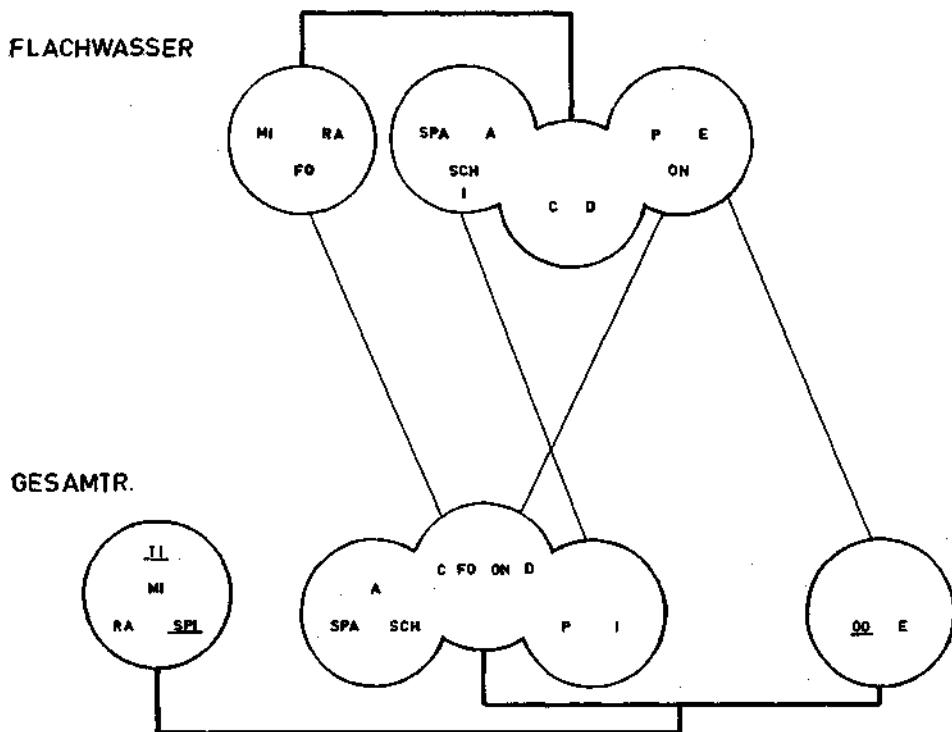
Abb. 7. Gegenüberstellung von Variablengruppen des Gesamttraumes und der Flachwasserkalke (vgl. Abb. 1).
