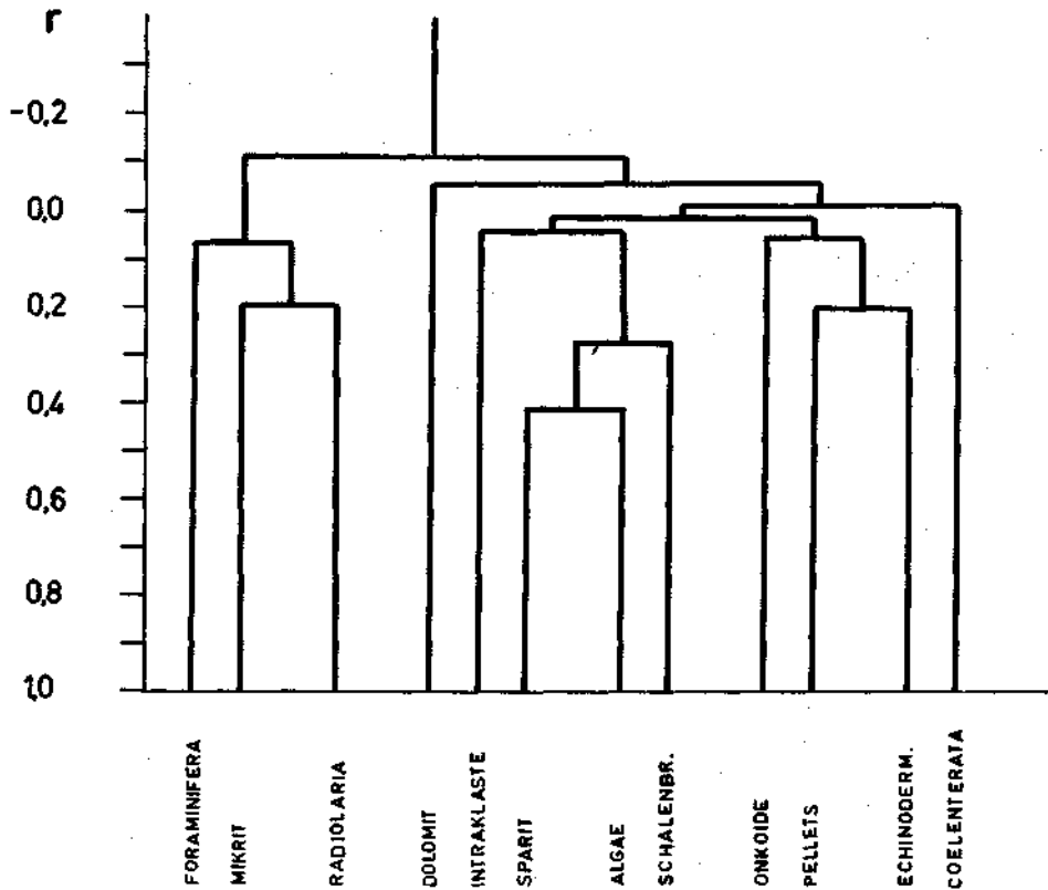
Abb. 6. R-mode Clusterdiagramm für 12 Variable der Flachwasserkalke. Fig. 6. R-mode cluster diagram for 12 variables of the shallow water limestones.
