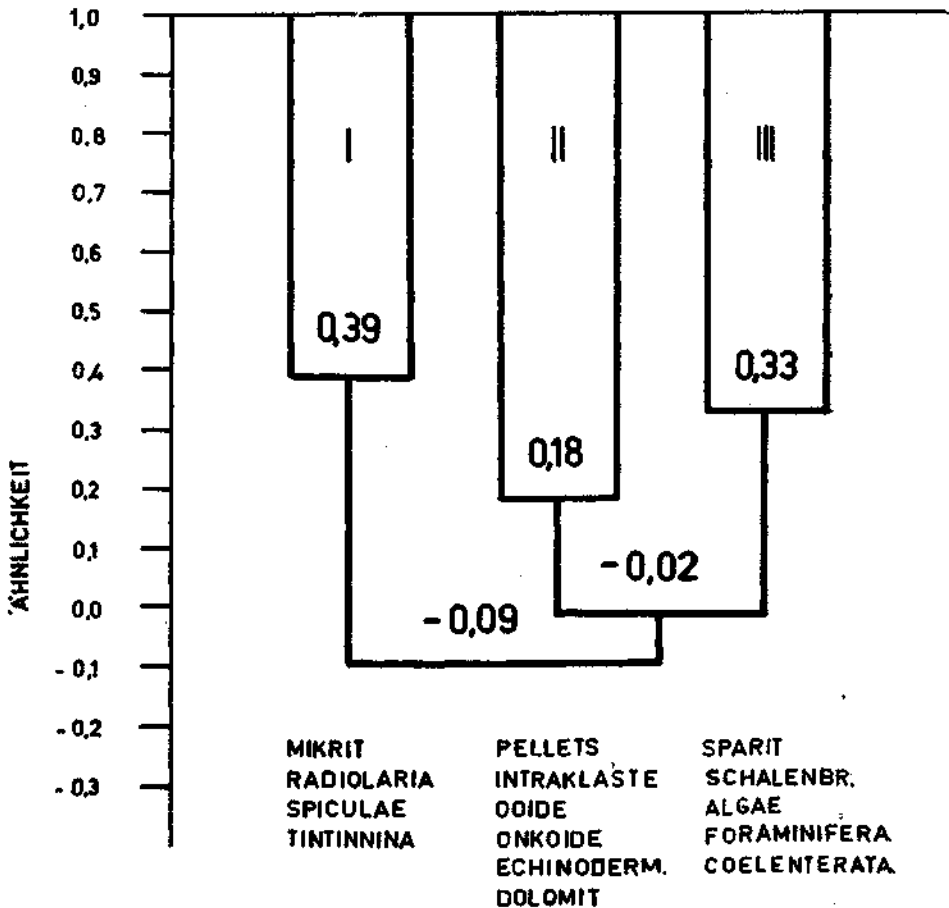
Abb. 4. Clusterdiagramm der 3 R-mode „factor reaction groups“ (bezogen auf Variable des Gesamttraumes).
