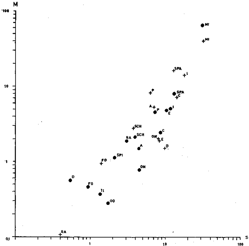
Abb. 1. Mittelwert gegen Standardabweichung.
