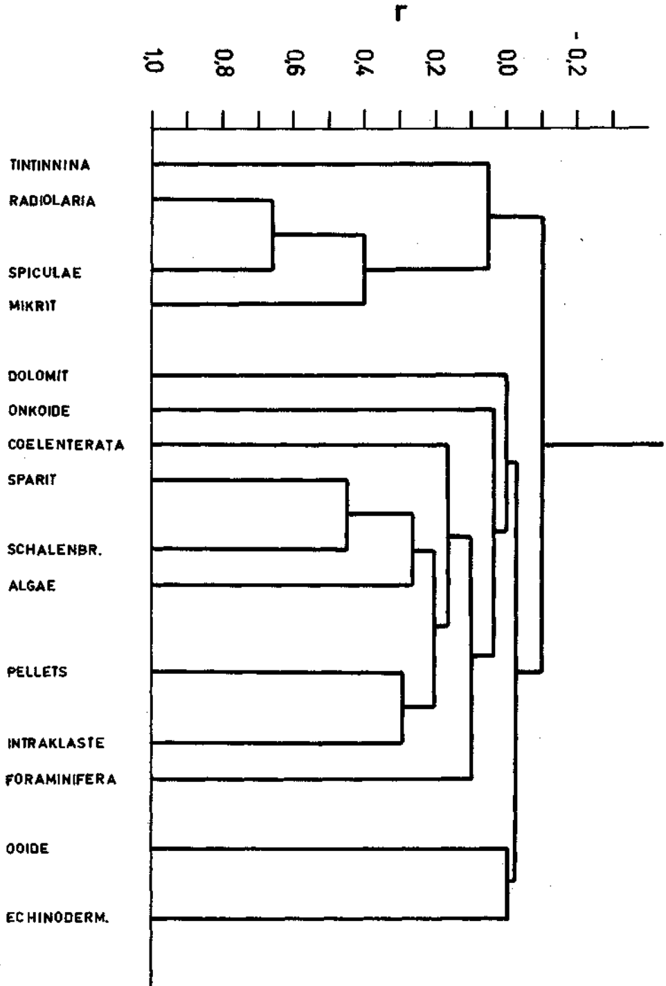
Abb. 3. R-mode Clusterdiagramm für 15 Variable (WVGMA). Fig. 3. R-mode cluster diagram for 15 variables (WVGMA).
