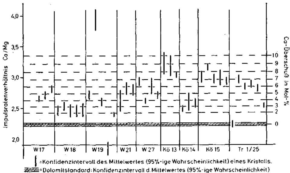
Abb. 1. Mit der Elektronenstrahl-Mikrosonde gemessene Ca-Mg-Verhältnisse spät-diagenetisch gebildeter Dolomitenkristalle. W 17, W 18 usw. sind Probenbezeichnungen.
