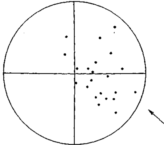
Abb. 2. Lage der Wachstumszentren der Dolomickörner in den verdrängten Ooiden (Dünnschliff Nr. 2512, vgl. Taf. II, Fig. 7). Der Pfeil zeigt die wahrscheinliche Strömungsrichtung der Dolomitisierungslösungen.
