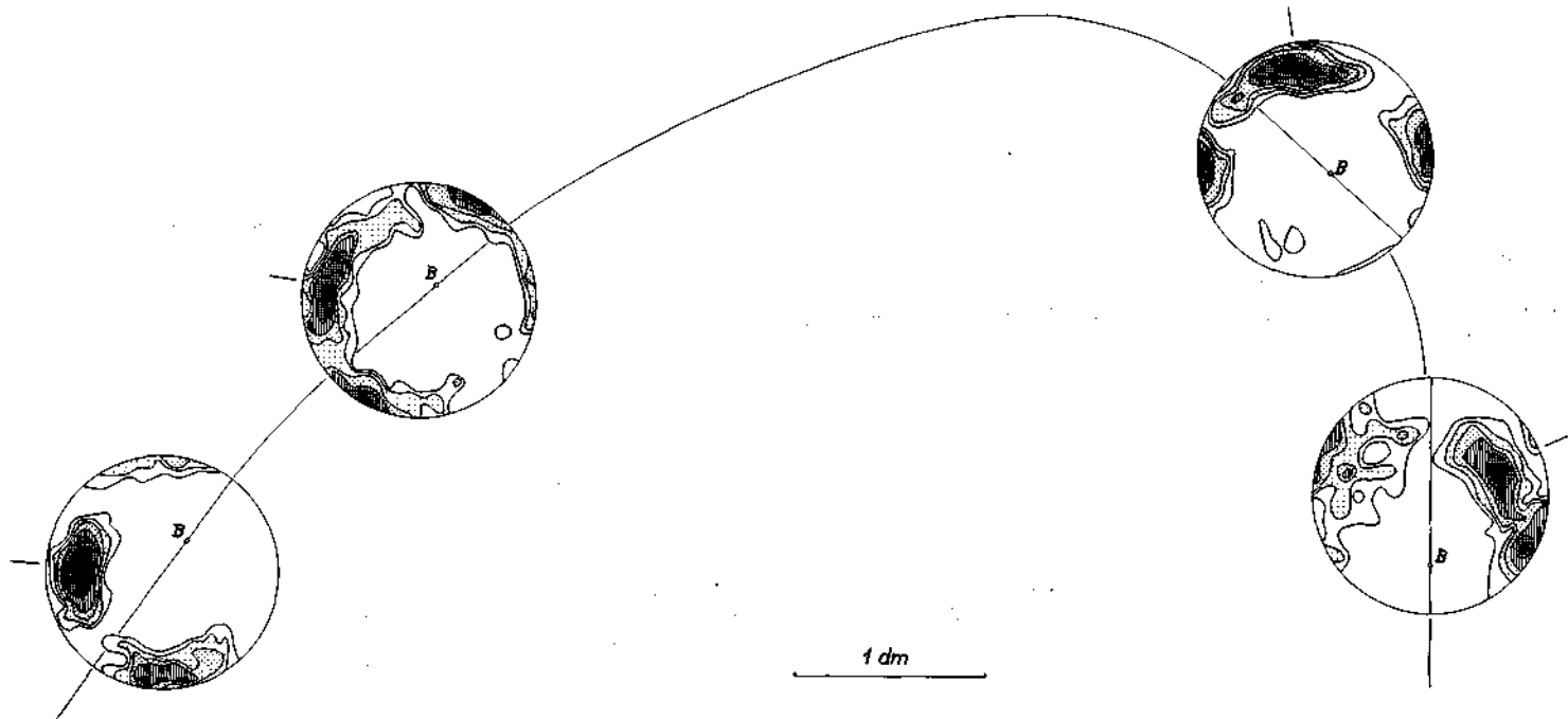
Abb. 1: Querschnitt durch eine Falte im Quarzrit der äußeren Phyllite bei Koroužné, mit eingezeichneten Probeentnahmeorten. Die Quarzgefügediagramme sind in die Schnittebene rotiert. 160—270 Quarz-c-Achsen. 0,0—1—2—3,5—5,5—8,5%. Maximale Belegungsdichten 11,5—17,5%.
