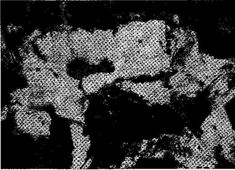
Abb. 2. Ortsbild aus der Baryt-Zonenvererzung. Baryt hellweiß, Nebengestein hellgrau. Deutlich erkennbar sind die im Baryt schwimmenden Dolomit-Nebengesteinsstücke. Letztere werden mit einem Saum von idiomorphen Fahlerzkristallen umgeben.
