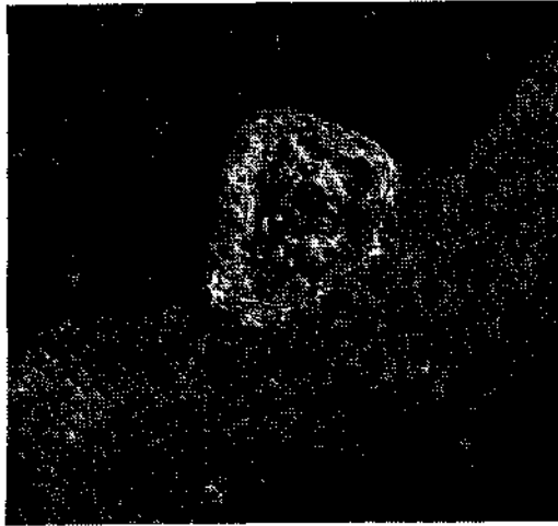
Fig. 1: Grenze zwischen Dachsteinkalk (hell) und Klaus-Schichten (dunkel). Korrosionsrelief durch Fe/Mn-reichen Rotkalk plombiert. Prielgraben; in natürlicher Größe.
