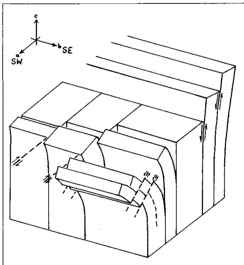
Abb. 7. Schema des Verformungsmechanismus.
